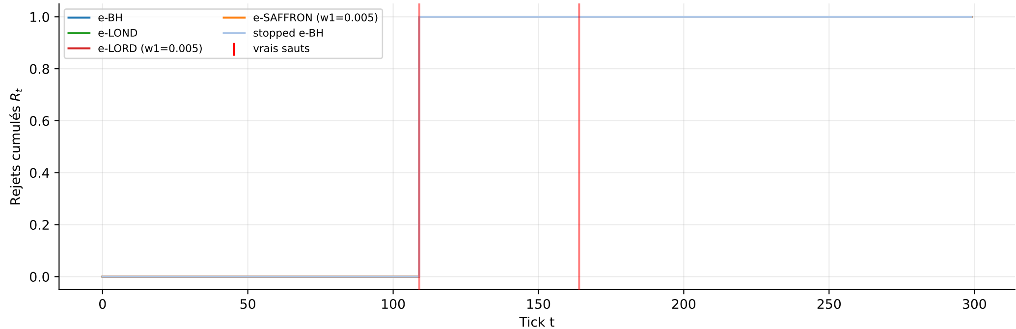
Rejets cumulés par algo — Heston+Merton moderate | n=300 , \alpha=0.05
