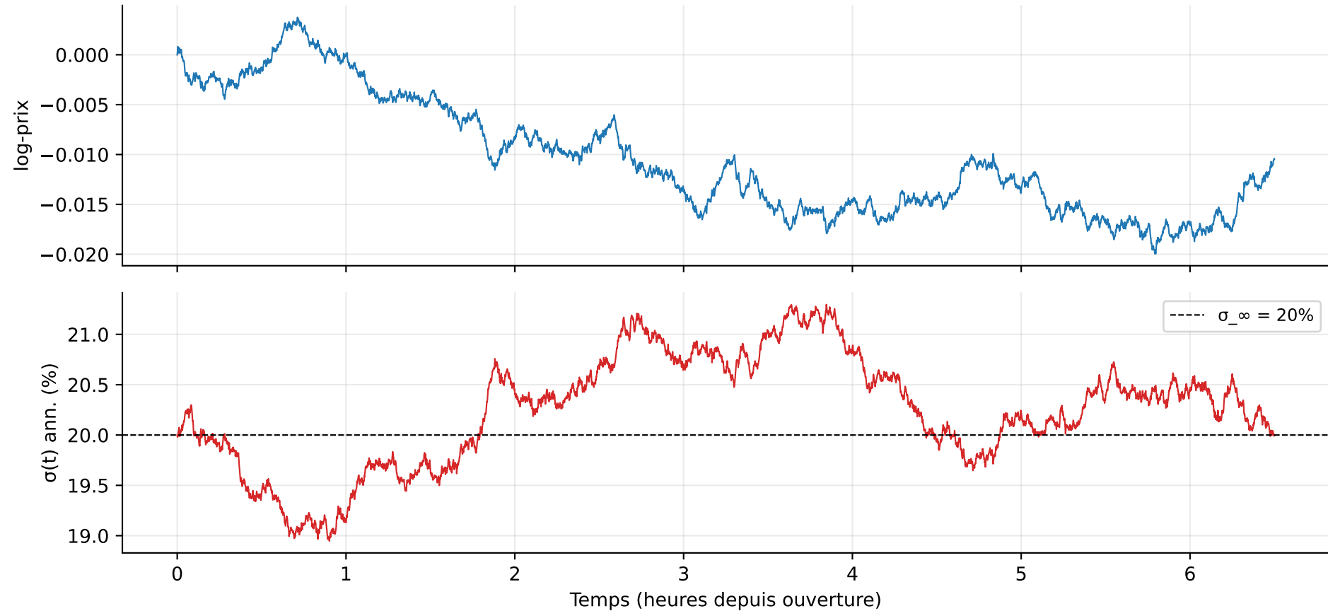
Heston pur — Schéma QE (Andersen 2008) | 1 journée à dt=5s
