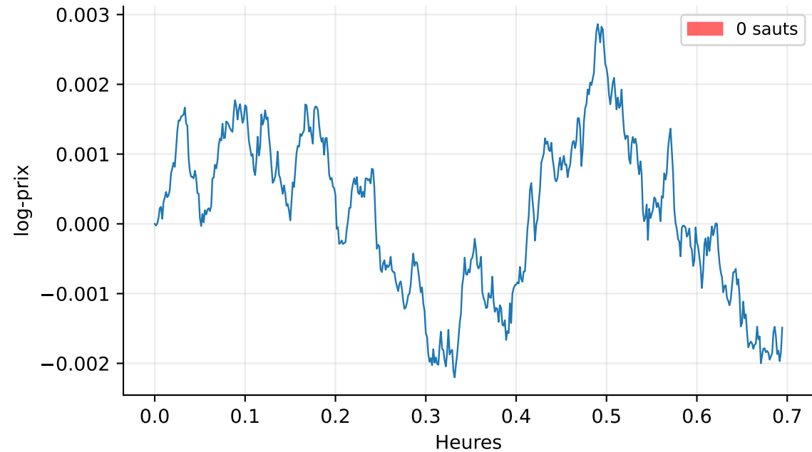
Heston+Merton ( \lambda=5000/\text{an} , \text{taille}=0.00092 ) 0 sauts en 0.7h
