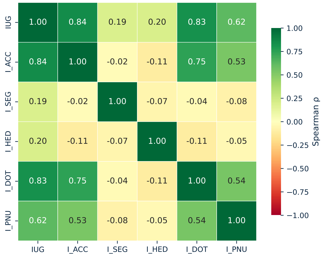
Correlación de Spearman
