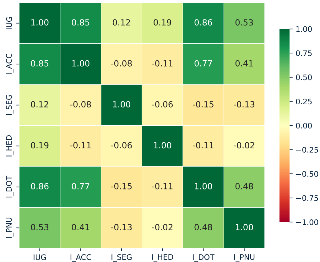
Correlación de Pearson
