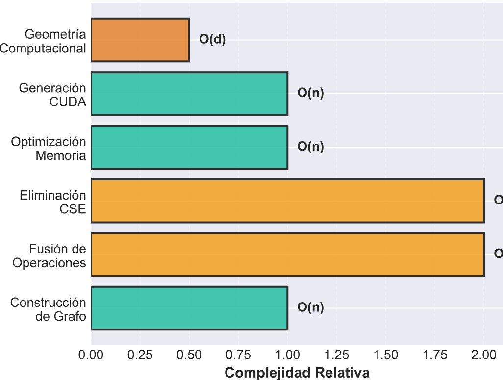
Complejidad de Algoritmos Implementados
