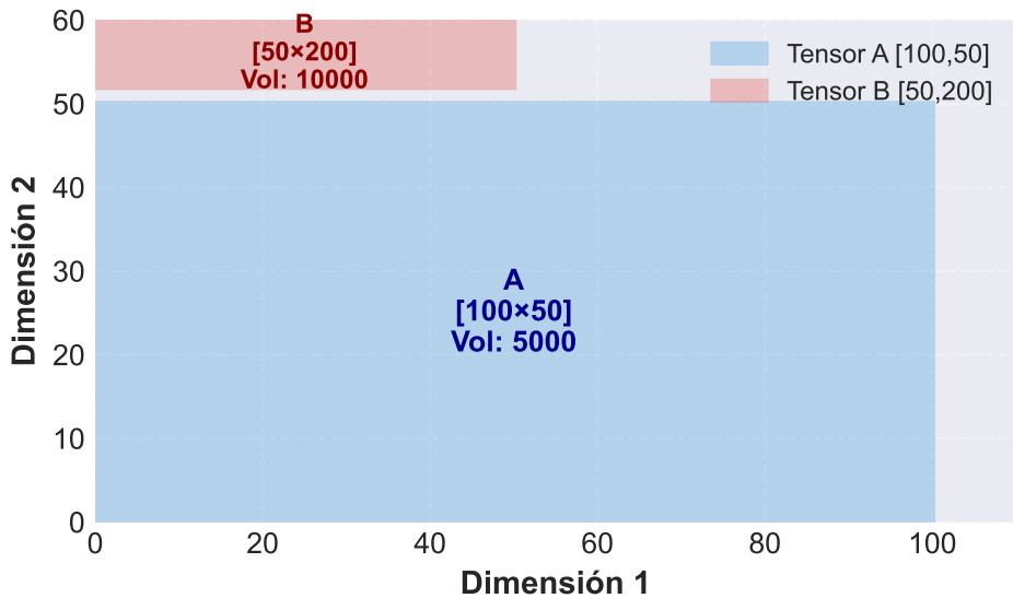
Espacios de Iteración de Tensores
