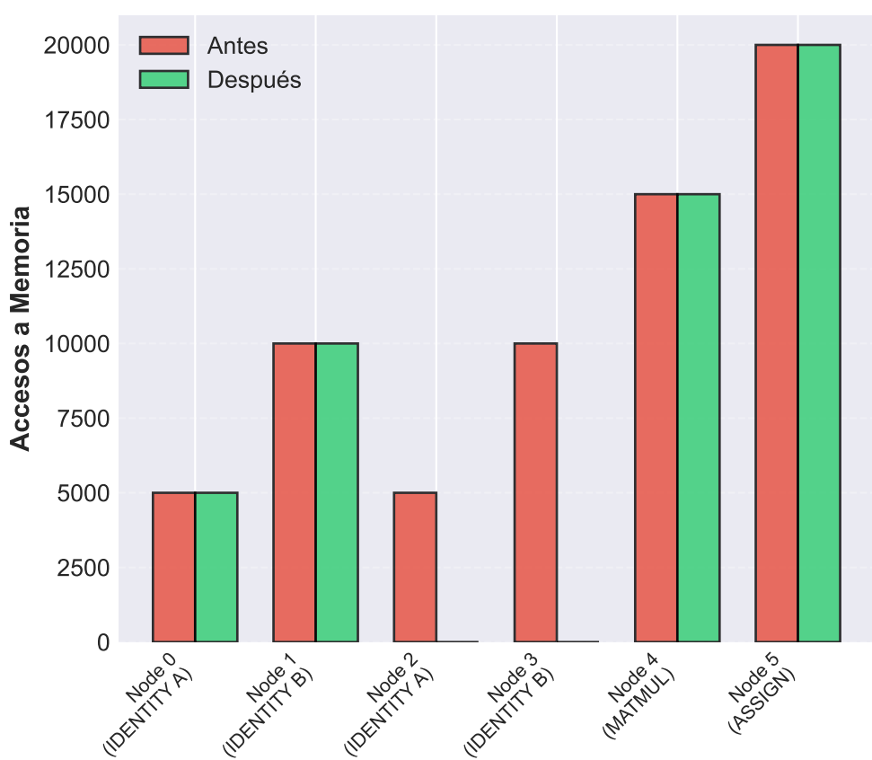
Accesos a Memoria por Nodo
