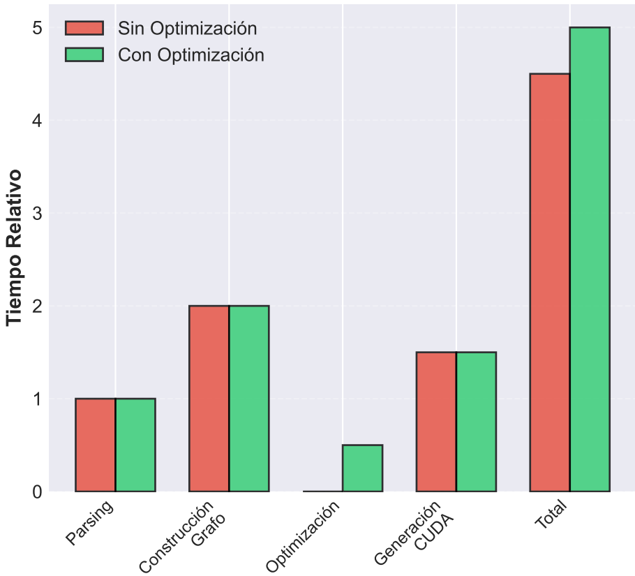
Tiempo de Compilación por Fase
