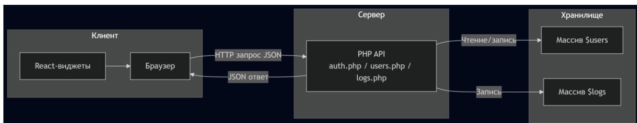
Скриншот 2 - Схема архитектуры (браузер <-> PHP API <-> массив).
