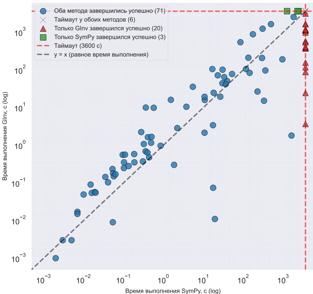
Диаграмма рассеяния времени вычисления базиса Грёбнера при использовании различных типов полиномиального деления
