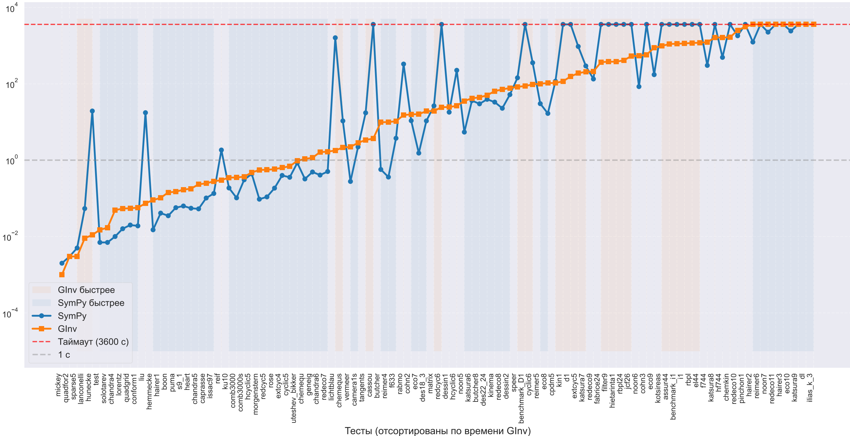
Сравнение времени вычисления базиса Грёбнера в библиотеках SymPy и GInV (с сортировкой по времени GInV)
