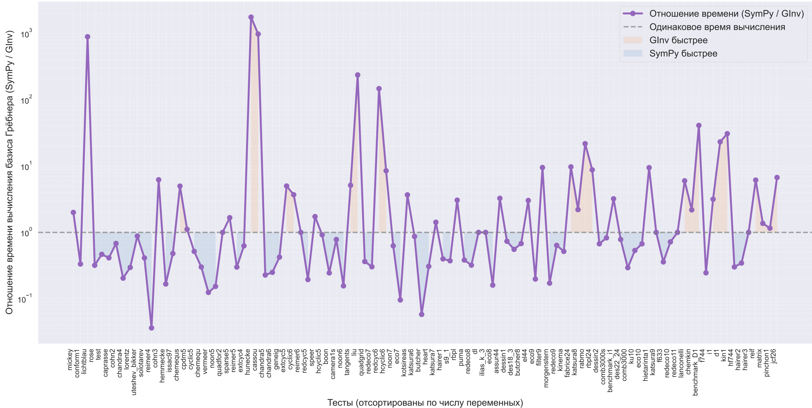
Отношение времени вычисления базиса Грёбнера при использовании библиотек SymPy и GInV (с сортировкой по числу переменных)
