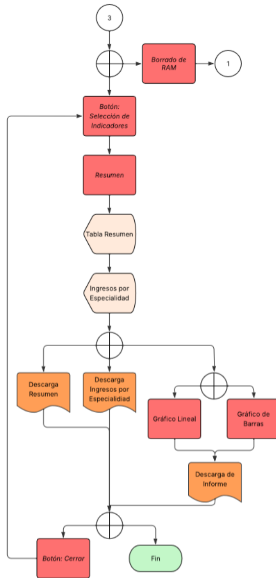
Figura B.6: Diagrama de flujo - Resumen.
