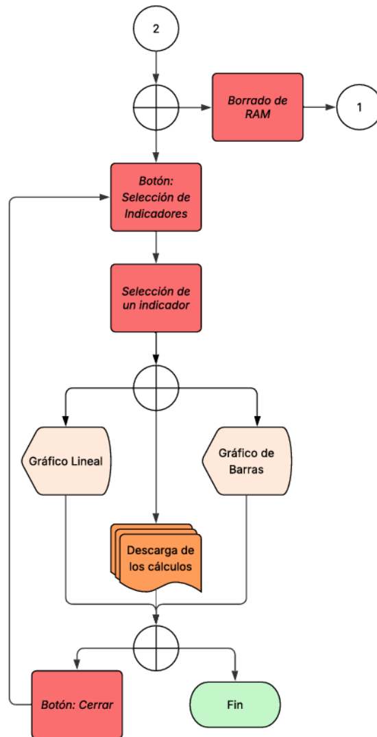
Figura B.5: Diagrama de flujo - Selección de indicadores.
