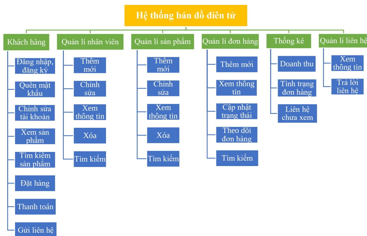
Hình 3.2 Sơ đồ phân rã chức năng.
