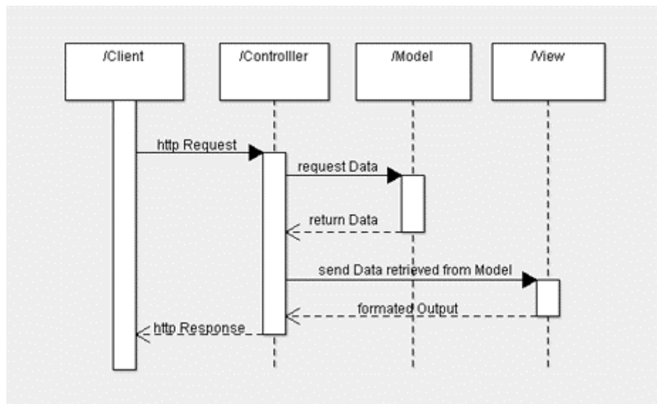
Hình 1.2. Mô hình tuần tự của MVC
