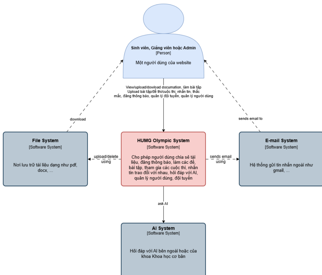
Hình 1. System Context
