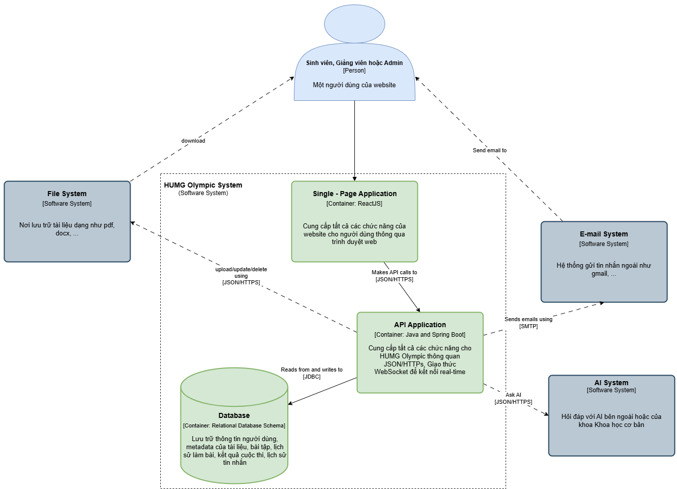
Hình 2. Container Diagram
