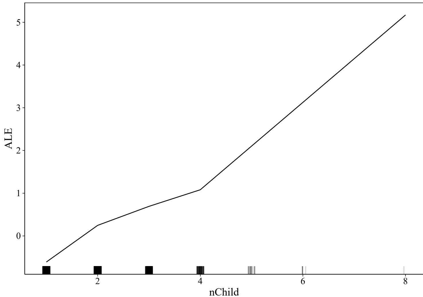
ALE plot: nChild
