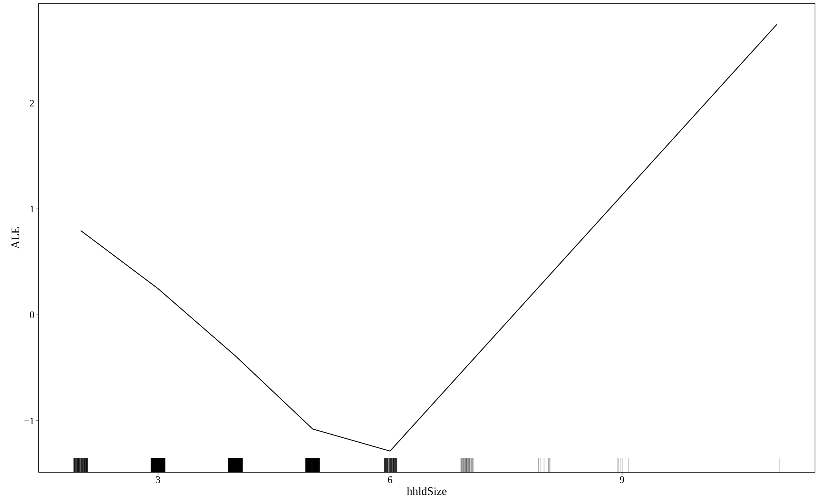
ALE plot: hhldSize
