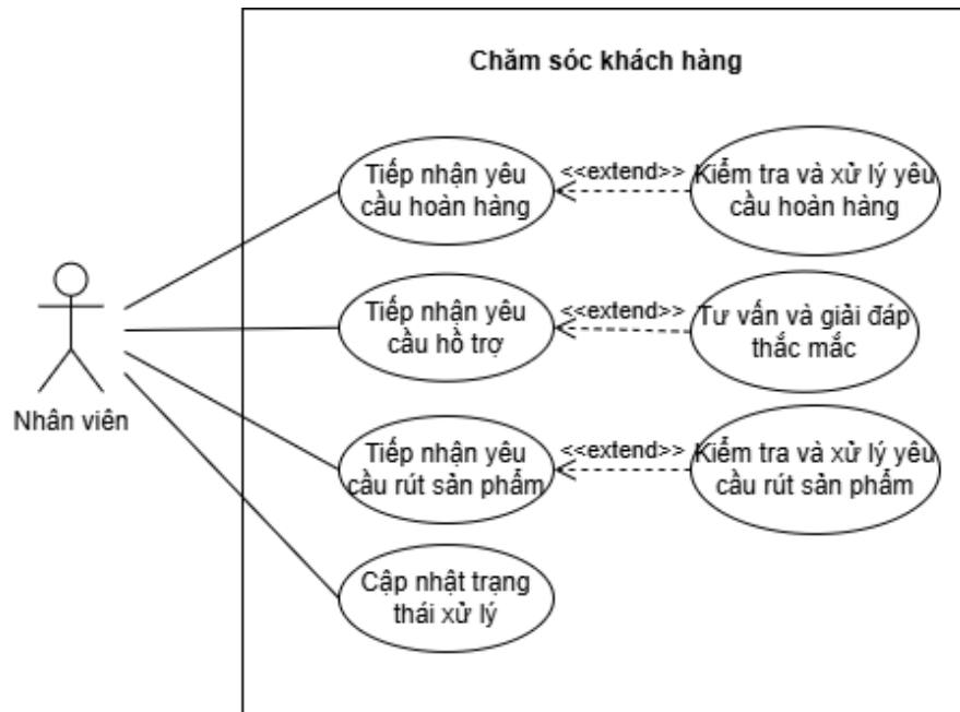
Hình 3.14: Sơ đồ use case phân rã cho use case Chăm sóc khách hàng
