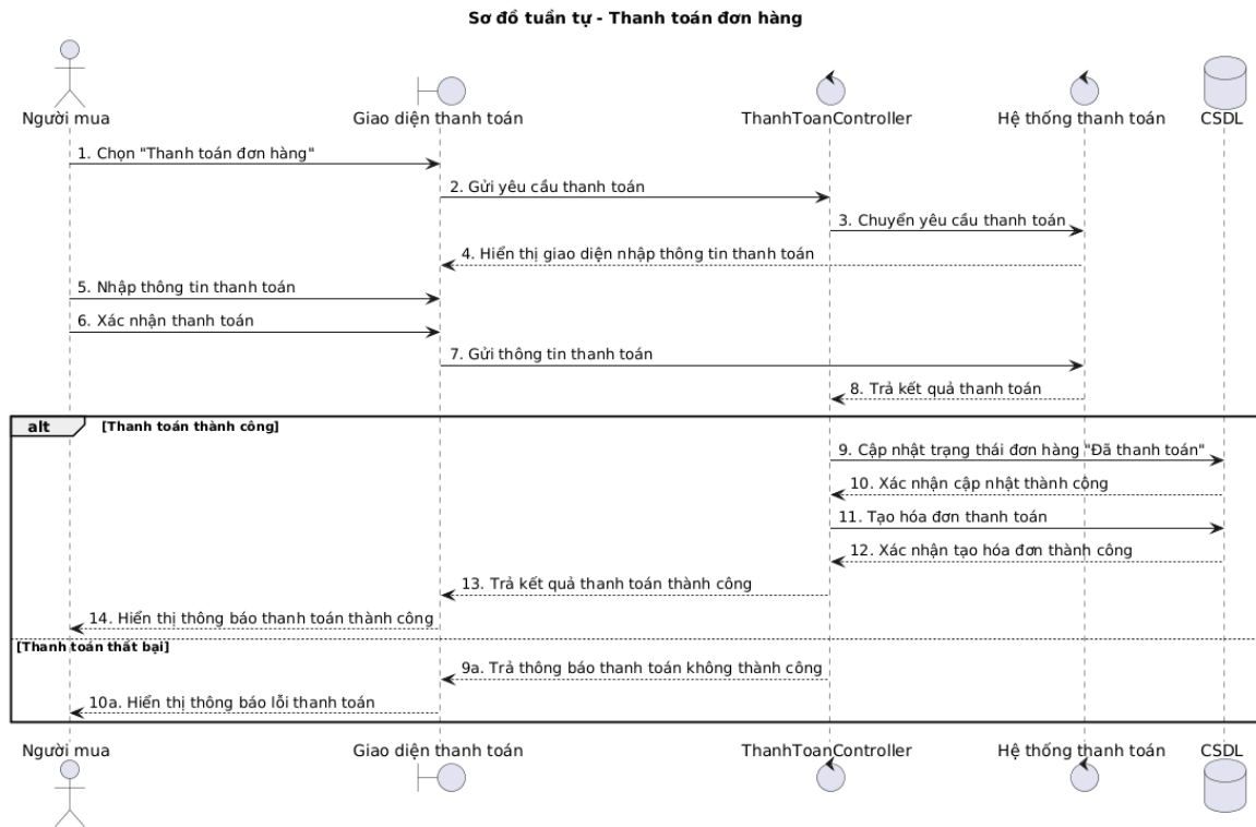
Hình 3.24: Sơ đồ tuần tự "Thanh toán"
