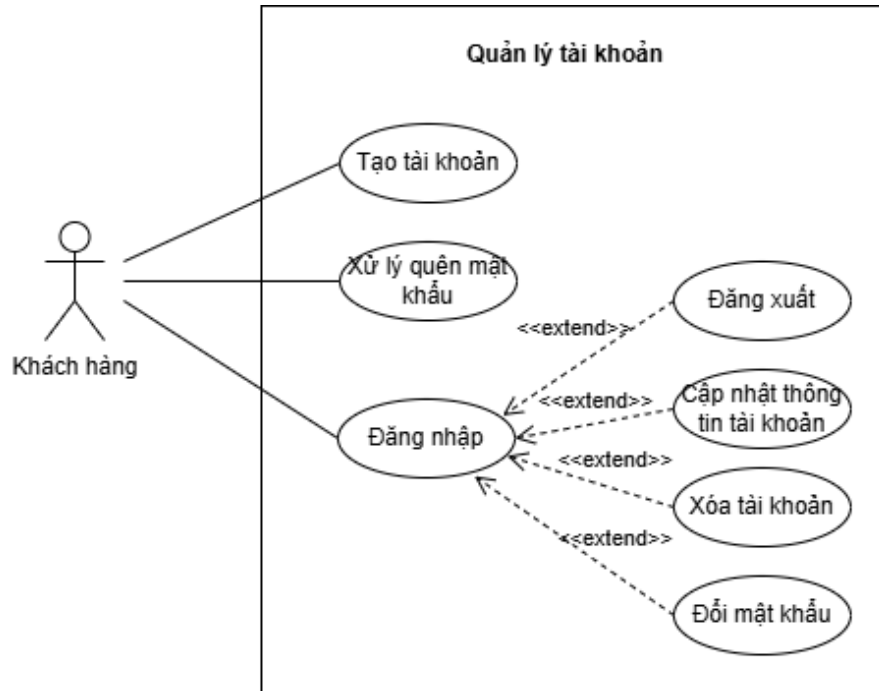
Hình 3.1: Sơ đồ use case phân rã cho use case Quản lý tài khoản
