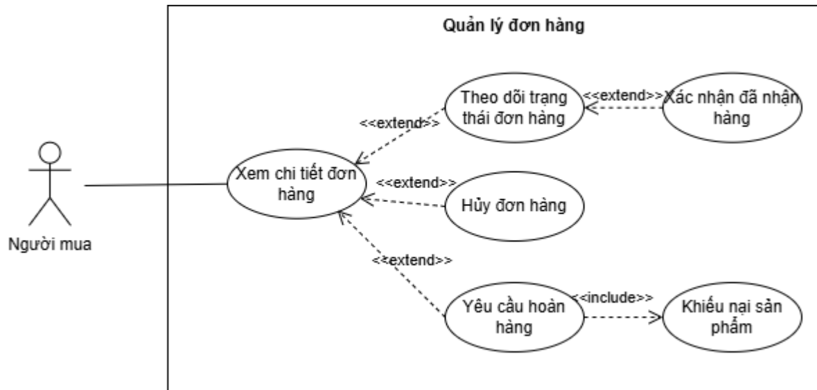
Hình 3.7: Sơ đồ use case phân rã cho use case Quản lý đơn hàng
