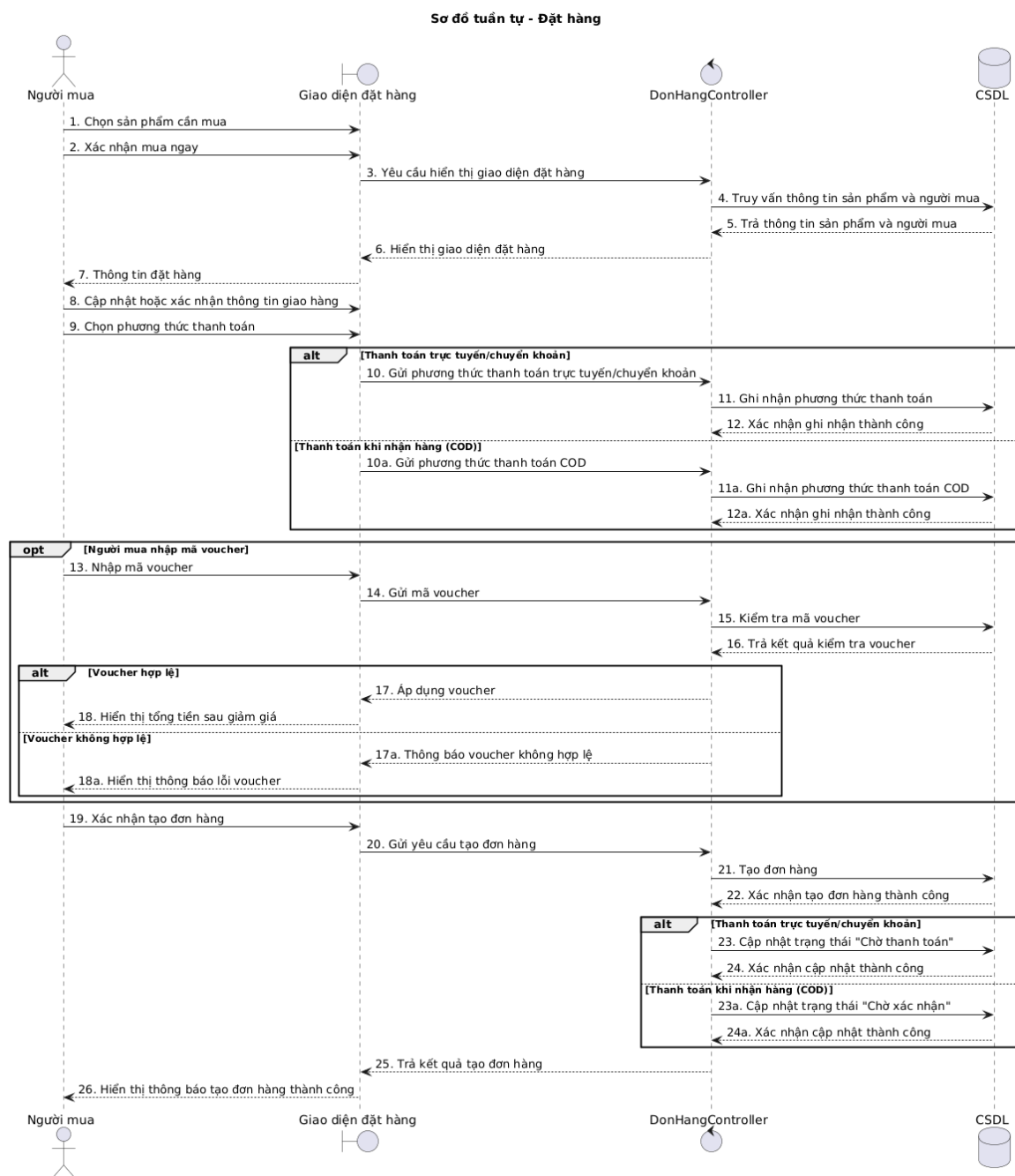
Hình 3.23: Sơ đồ tuần tự "Đặt hàng"
