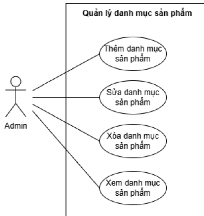
Hình 3.15: Sơ đồ use case phân rã cho use case Quản lý danh mục sản phẩm
