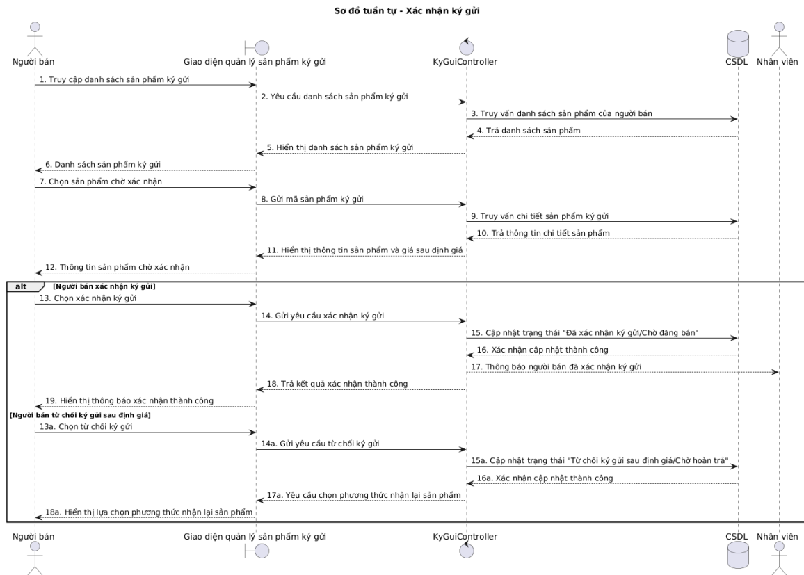
Hình 3.21: Sơ đồ tuần tự "Xác nhận ký gửi"
