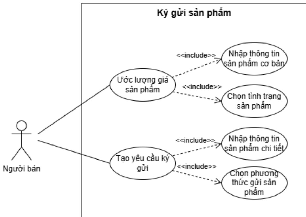
Hình 3.2: Sơ đồ use case phân rã cho use case Ký gửi sản phẩm
