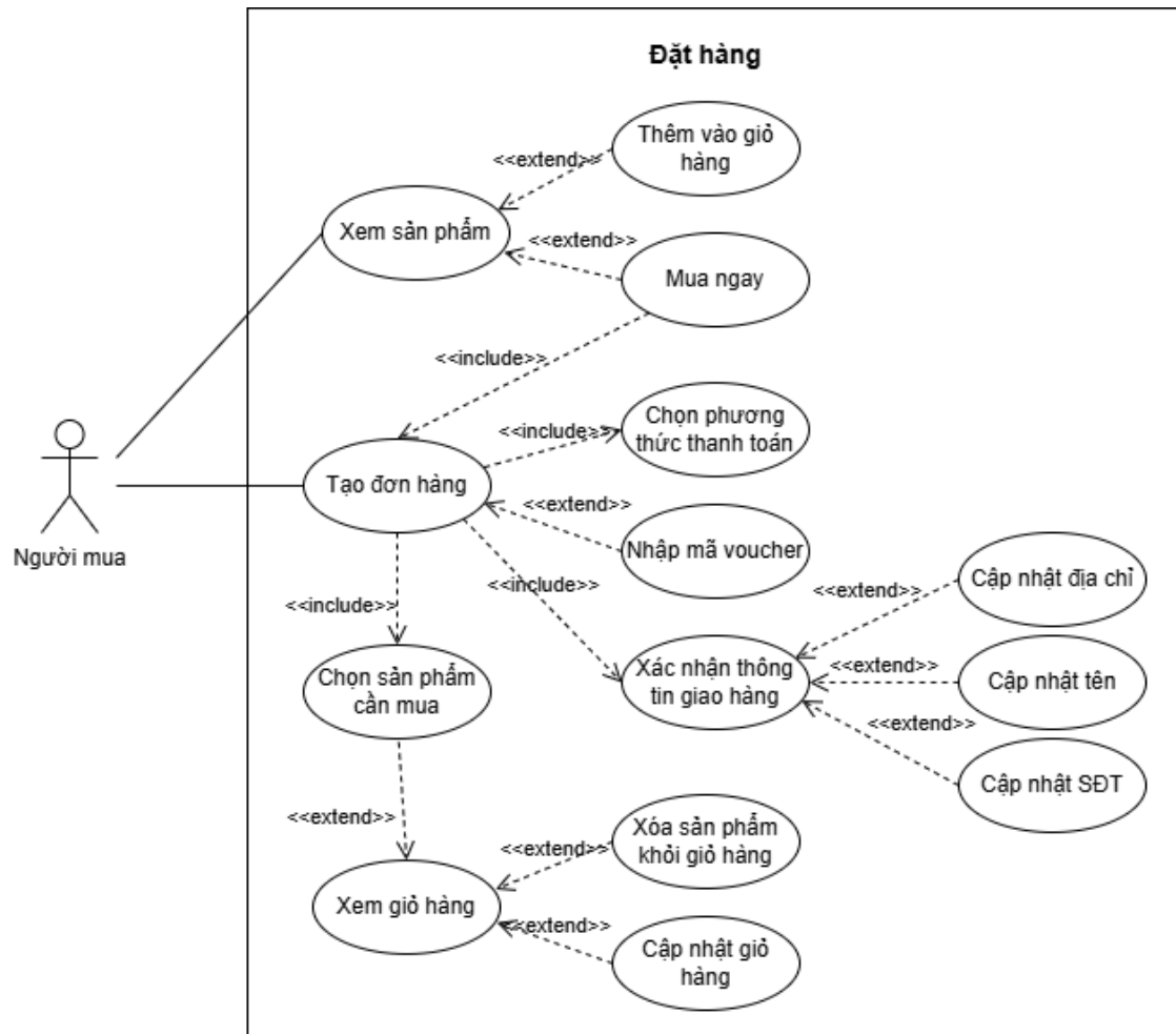
Hình 3.5: Sơ đồ use case phân rã cho use case Đặt hàng
