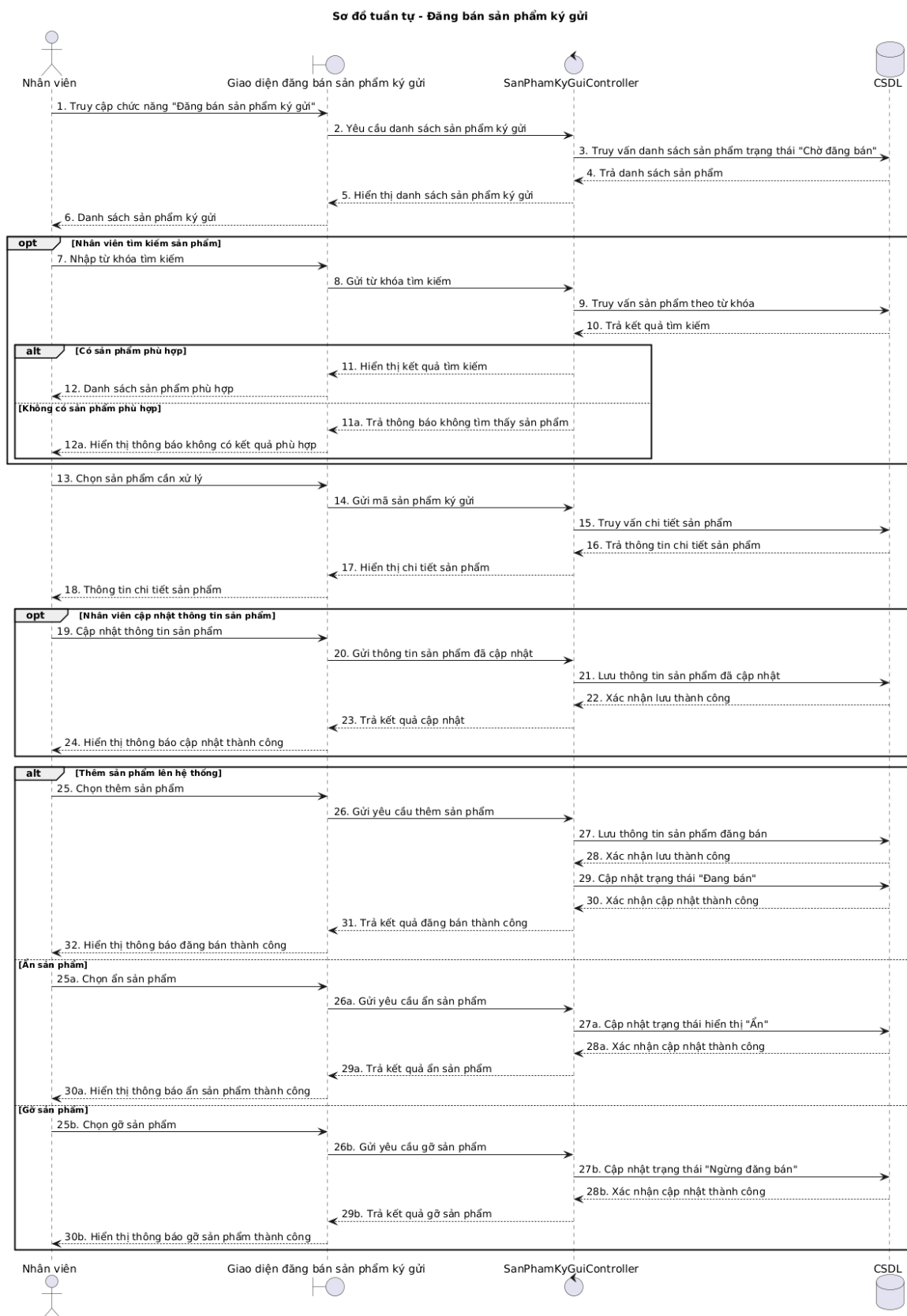
Hình 3.22: Sơ đồ tuần tự "Đăng bán sản phẩm ký gửi"
