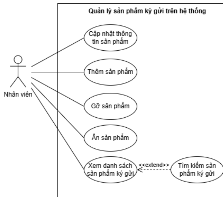
Hình 3.11: Sơ đồ use case phân rã cho use case Quản lý sản phẩm ký gửi trên hệ thống
