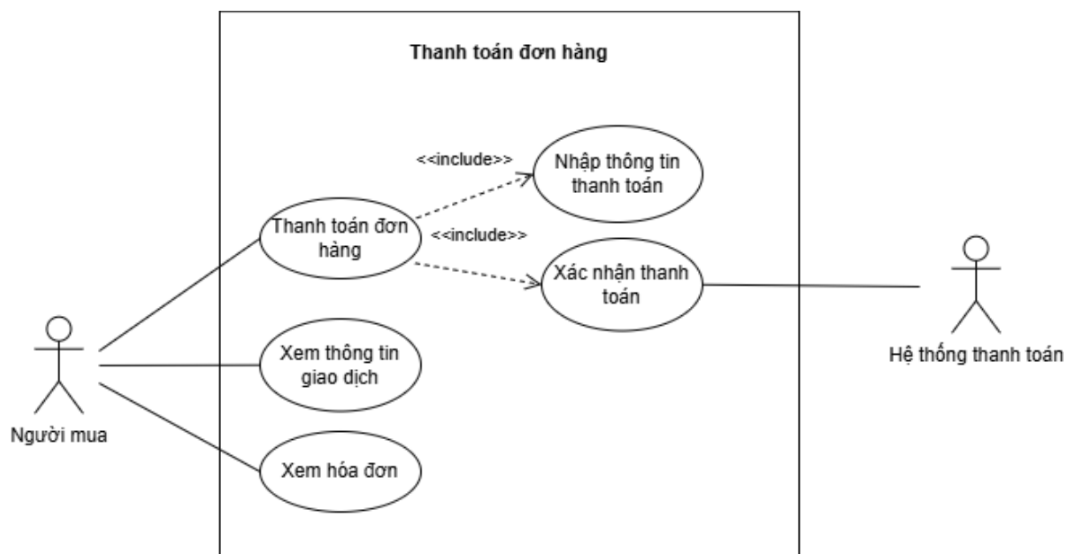
Hình 3.6: Sơ đồ use case phân rã cho use case Thanh toán đơn hàng
