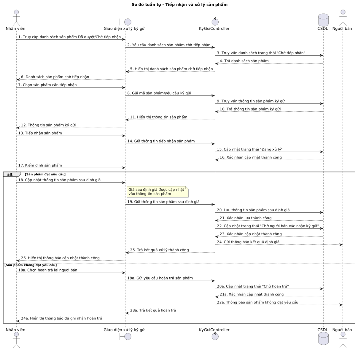
Hình 3.20: Sơ đồ tuần tự "Tiếp nhận và xử lý sản phẩm"
