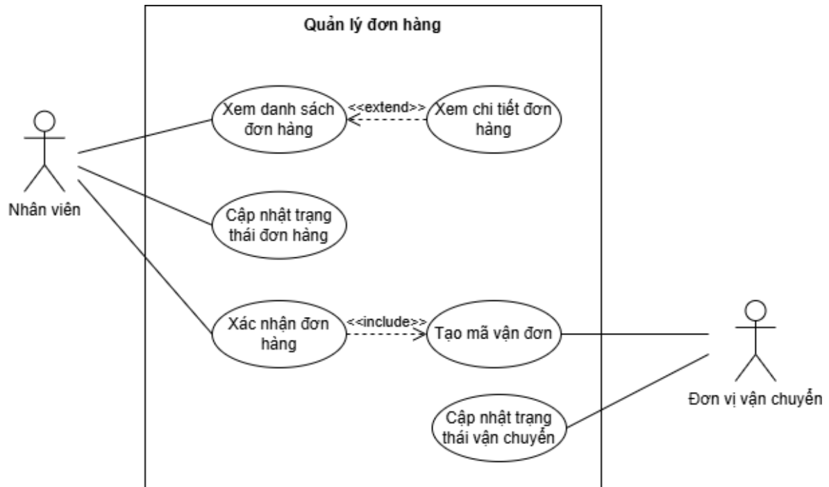
Hình 3.12: Sơ đồ use case phân rã cho use case Quản lý đơn hàng
