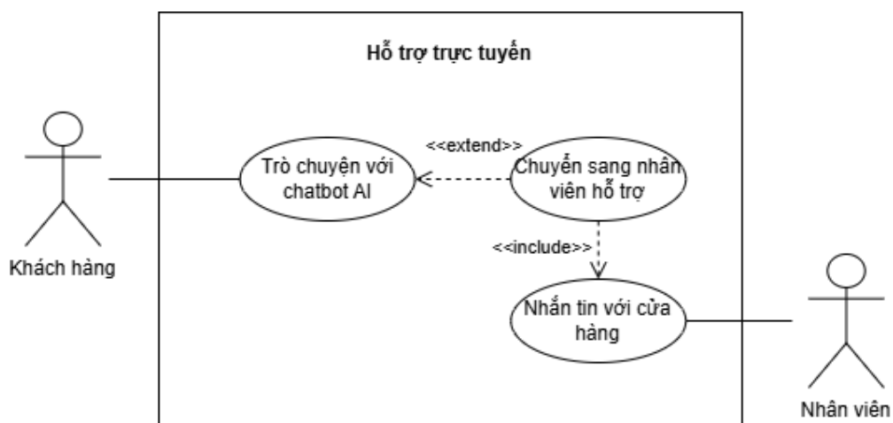
Hình 3.9: Sơ đồ use case phân rã cho use case Hỗ trợ trực tuyến
