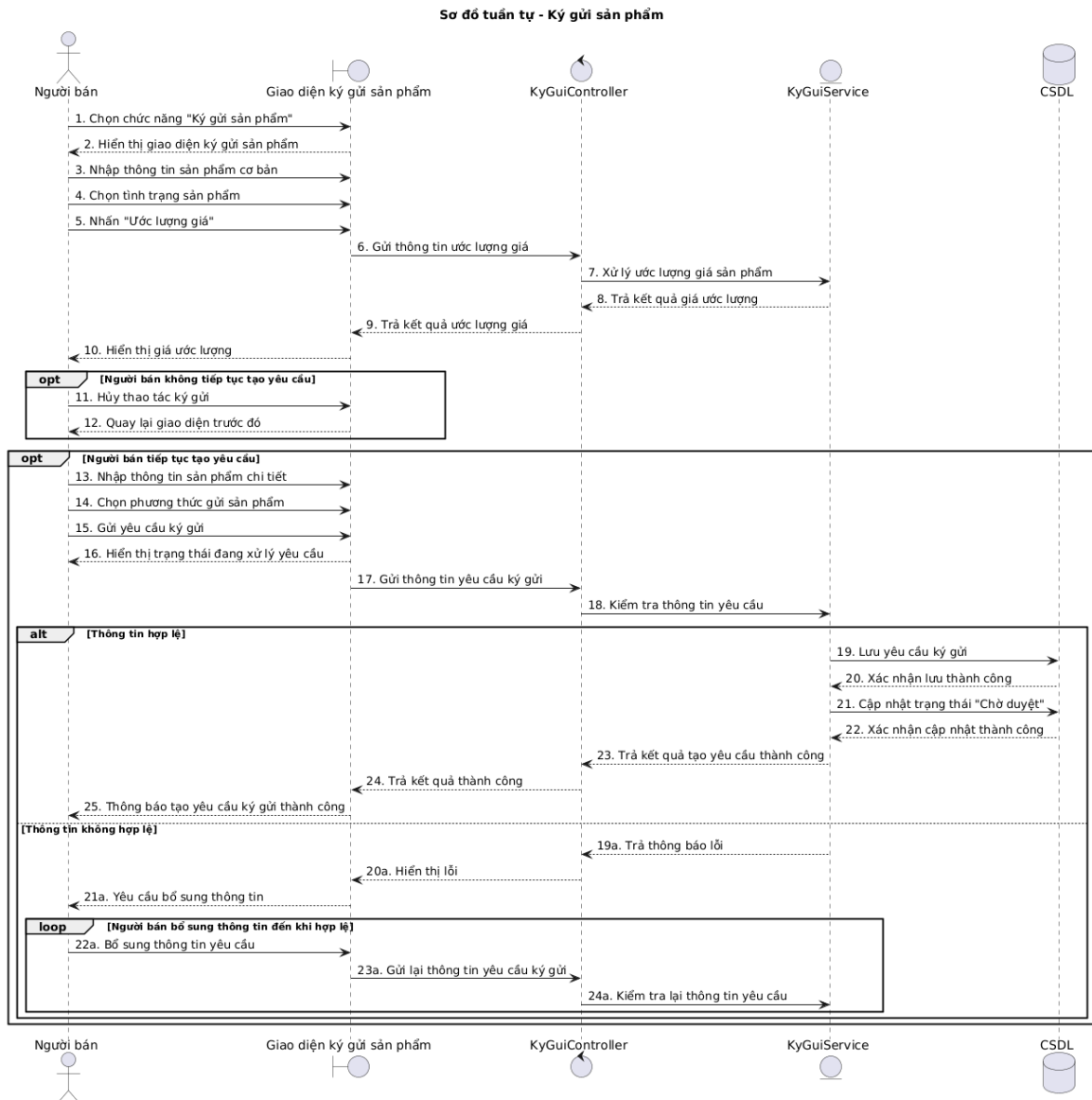
Hình 3.18: Sơ đồ tuần tự "Ký gửi sản phẩm"
