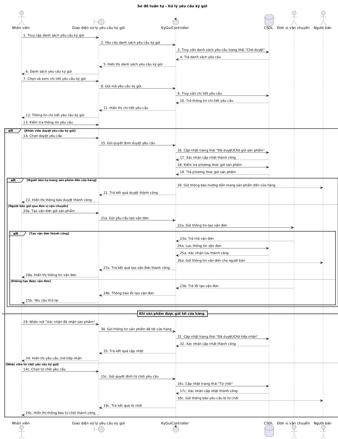
Hình 3.19: Sơ đồ tuần tự "Xử lý yêu cầu ký gửi"
