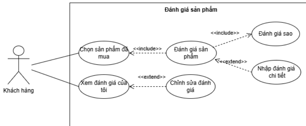
Hình 3.8: Sơ đồ use case phân rã cho use case Đánh giá sản phẩm
