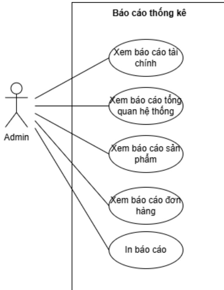
Hình 3.17: Sơ đồ use case phân rã cho use case Báo cáo thống kê
