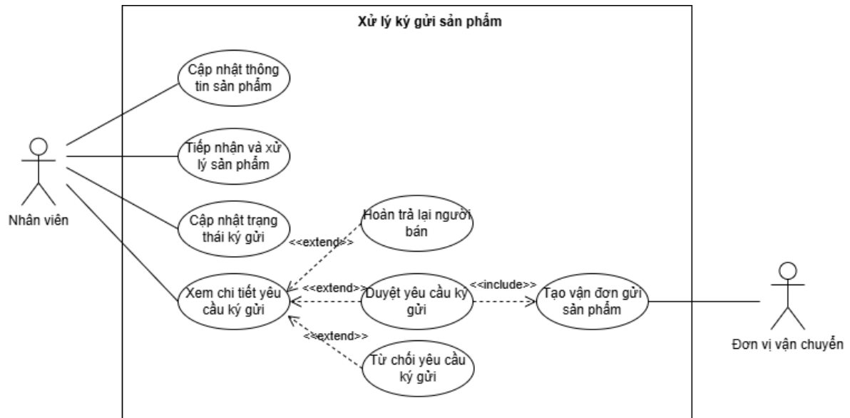
Hình 3.10: Sơ đồ use case phân rã cho use case Xử lý ký gửi sản phẩm
