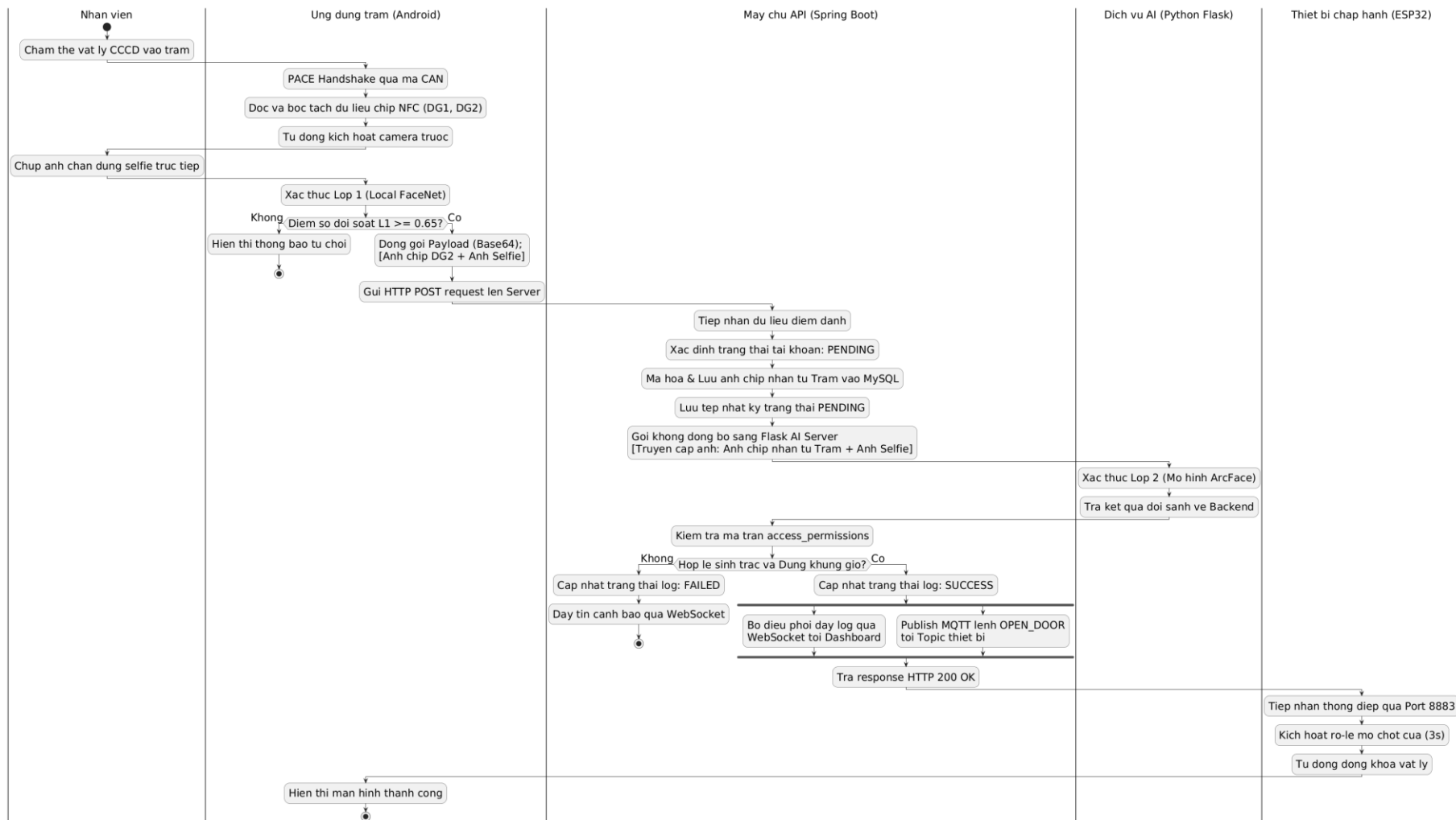
Sơ đồ hoạt động luồng Pending
