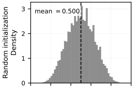
KDA
