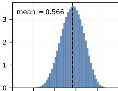
Isotropic KDN
