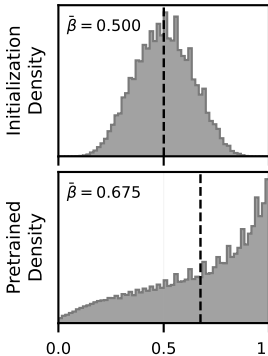
KDA
