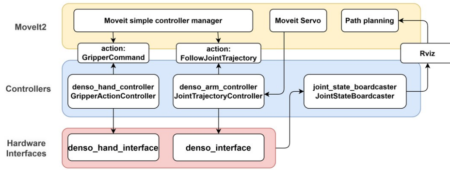
Hình 4.12: Sơ đồ khối Controllers trong kiến trúc Ros2-Control
