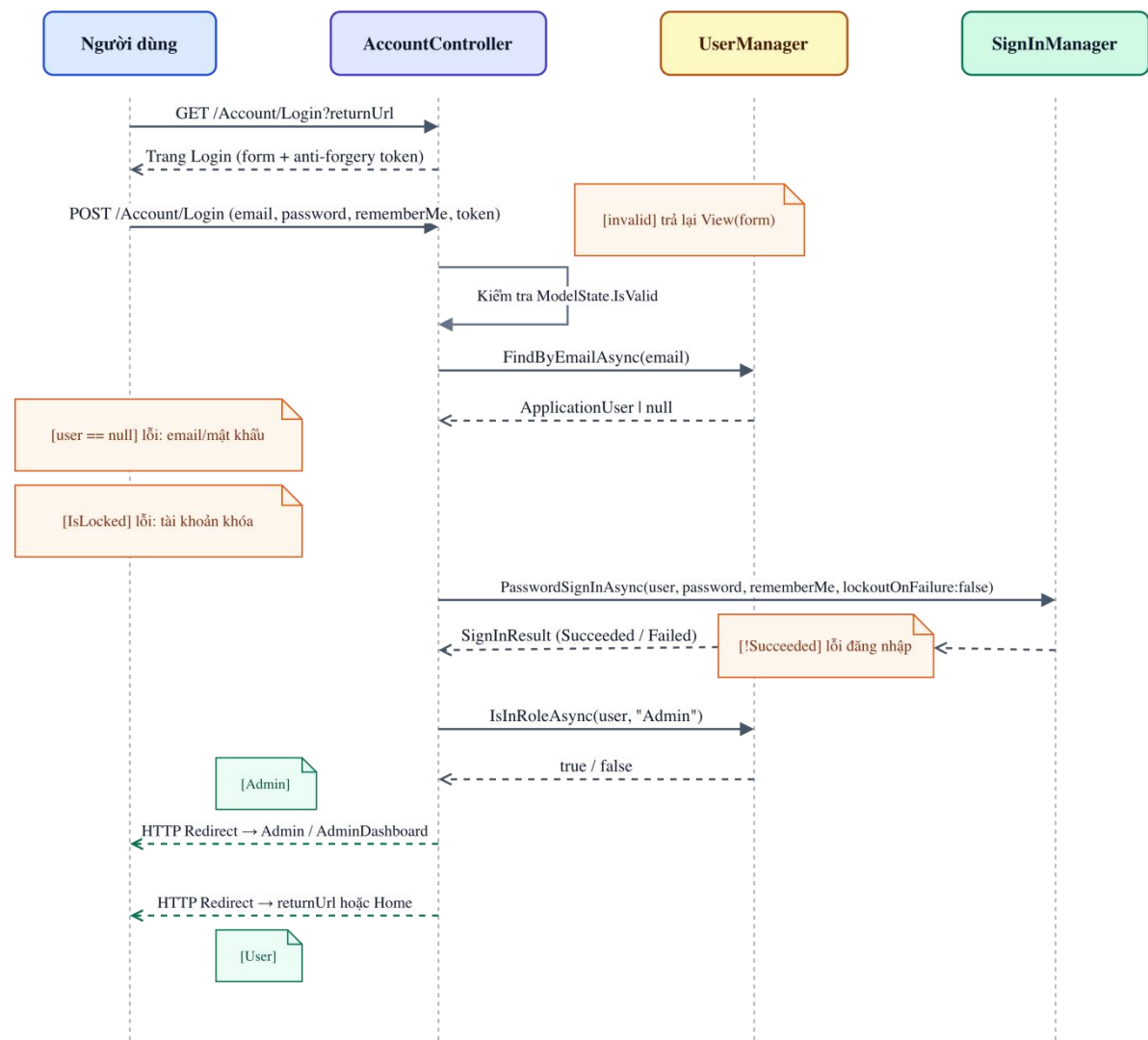
Sequence: Đăng nhập (AccountController.Login)
