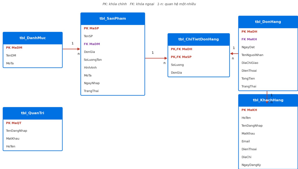
Hình 2.3. Mô hình dữ liệu quan hệ (ERD) của CSDL AppleStore
