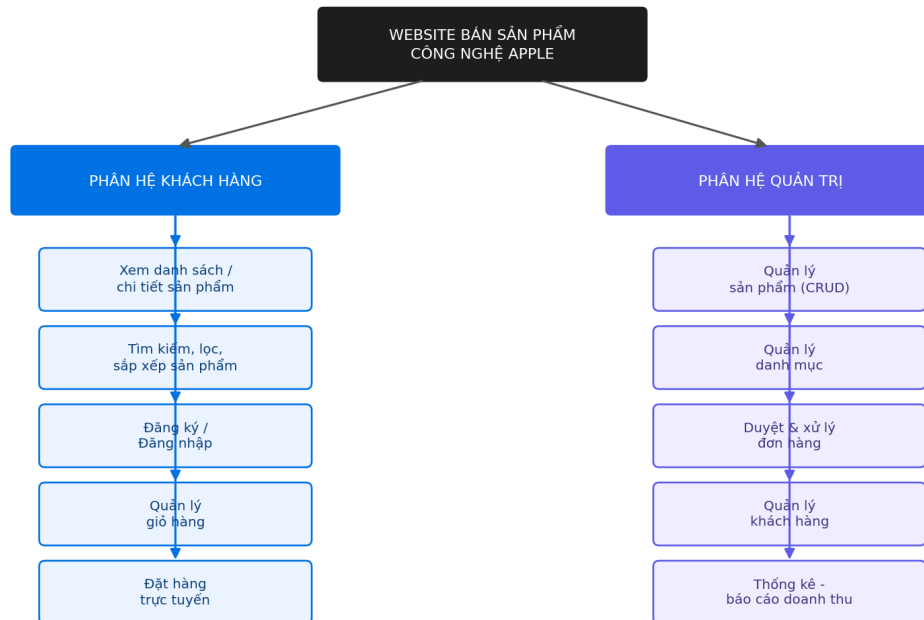
Hình 2.2. Sơ đồ phân rã chức năng của hệ thống
