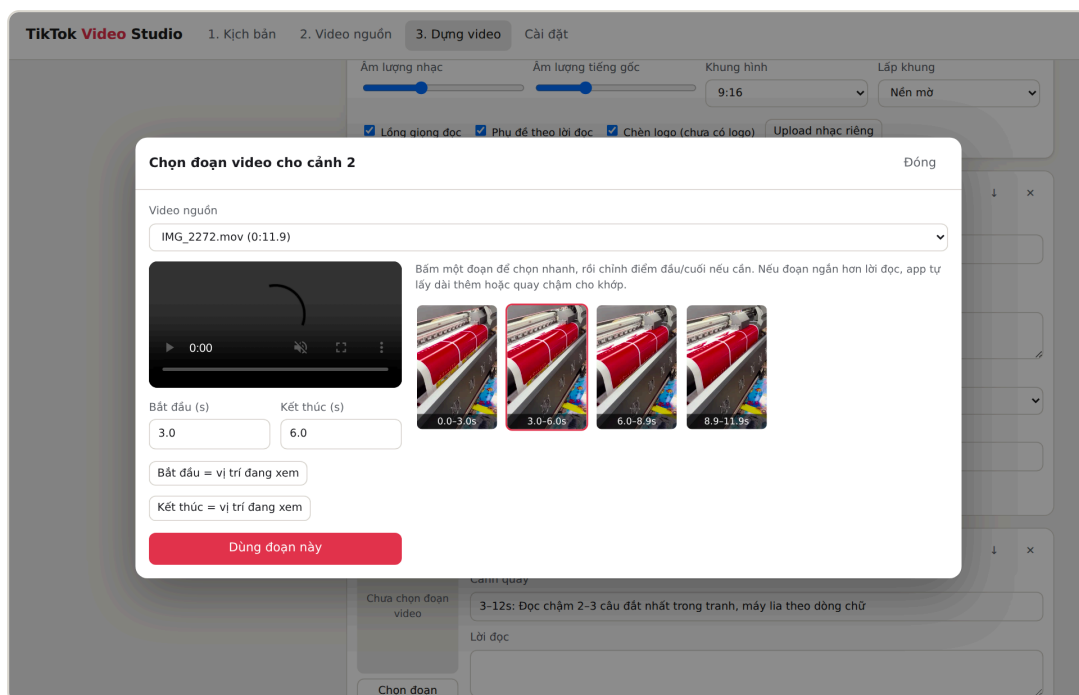
Hình 6. Hộp chọn đoạn video: bấm một ảnh đoạn (viền đỏ) rồi bấm “Dùng đoạn này”.
