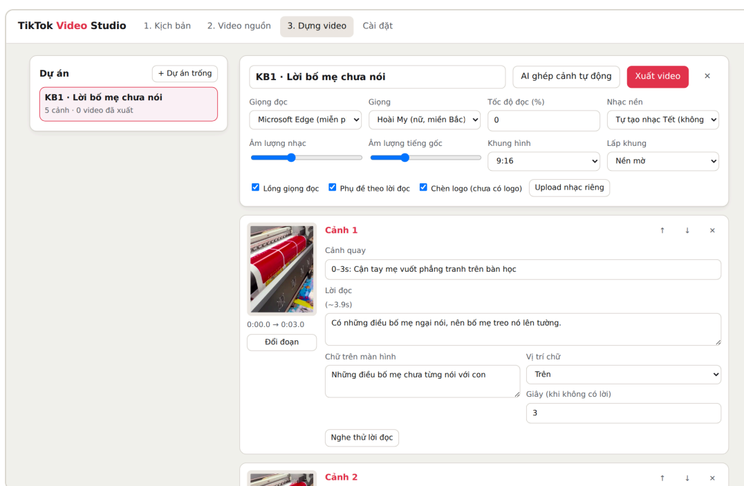
Hình 10. Tab Dụng video. Thanh trên cùng là nút AI ghép cảnh, Xuất video và các lựa chọn giọng đọc, nhạc, khung hình; bên dưới là từng cảnh.
