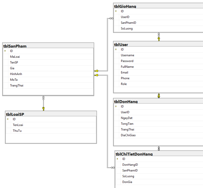
Bảng: sơ đồ Diagram kết nối giữa các bảng trực tiếp từ SQL Server
