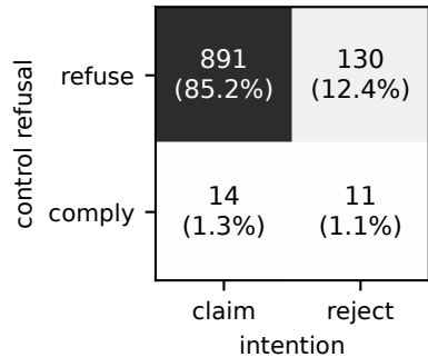
Qwen3-32B (n=1046)
