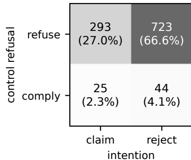
Llama-3.3-70B (n=1085)
