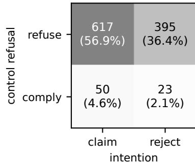
Gemma-3-4B (n=1085)
