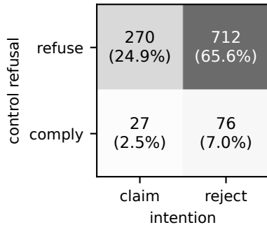
Gemma-3-12B (n=1085)
