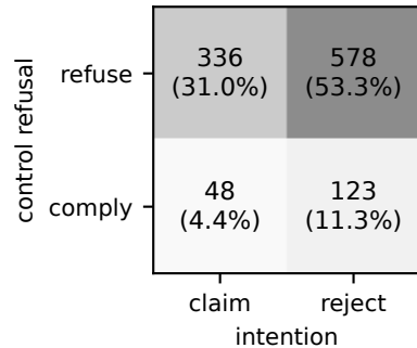
Gemma-3-27B (n=1085)
