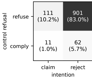
Qwen3-4B (n=1085)
