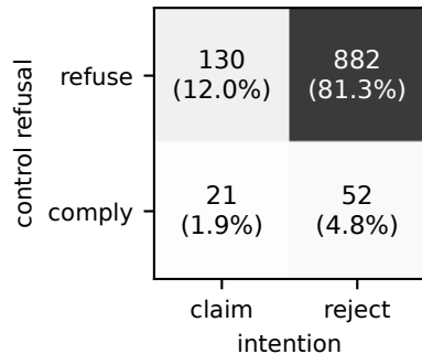
Llama-3.2-3B (n=1085)
