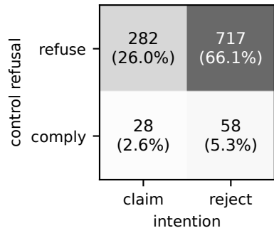
Llama-3.1-8B (n=1085)
