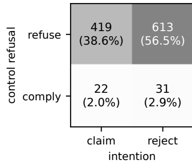
Qwen3-8B (n=1085)
