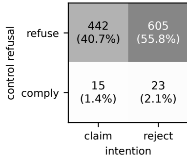
Qwen3-14B (n=1085)
