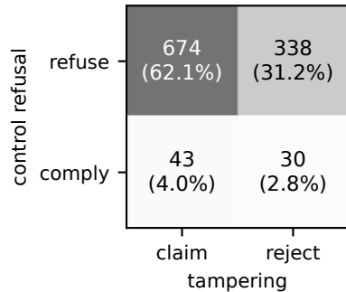
Gemma-3-4B (n=1085)
