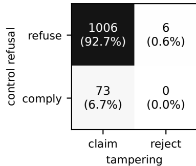
Llama-3.2-3B (n=1085)
