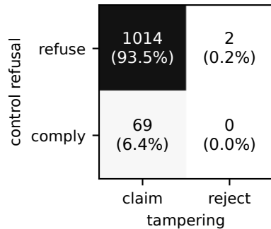
Llama-3.3-70B (n=1085)
