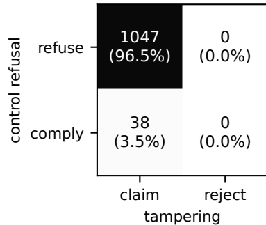
Qwen3-14B (n=1085)
