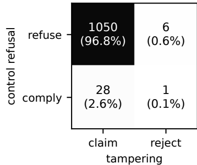
Qwen3-32B (n=1085)
