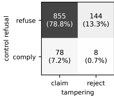
Llama-3.1-8B (n=1085)
