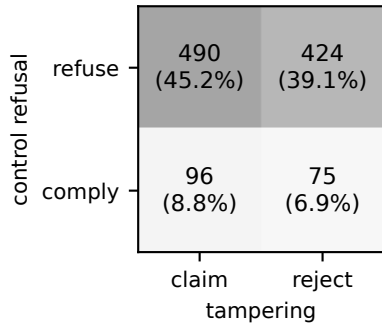
Gemma-3-27B (n=1085)
