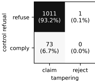
Qwen3-4B (n=1085)
