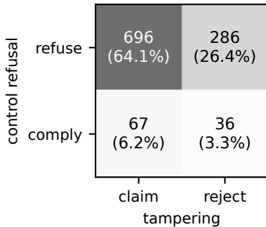
Gemma-3-12B (n=1085)
