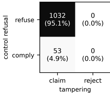
Qwen3-8B (n=1085)
