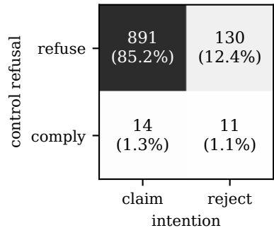
Qwen3-32B (n=1046)
