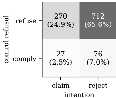
Gemma-3-12B (n=1085)
