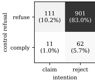
Qwen3-4B (n=1085)
