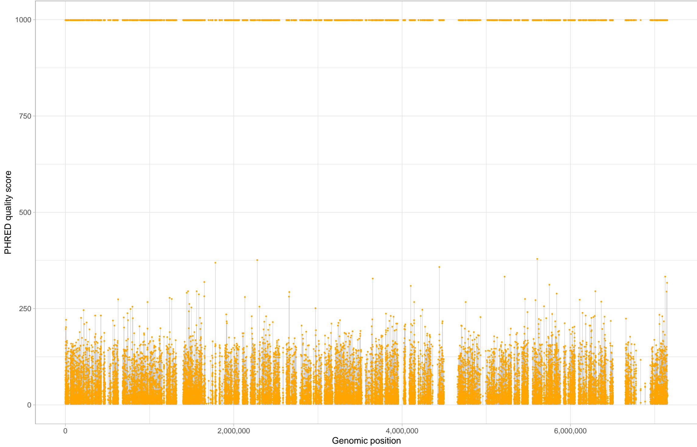
Chromosome chrZ
