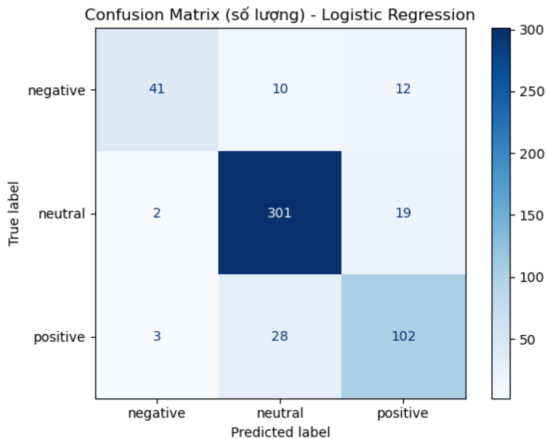
Hình 4.4.1: Confusion Matrix theo số lượng – Logistic Regression
