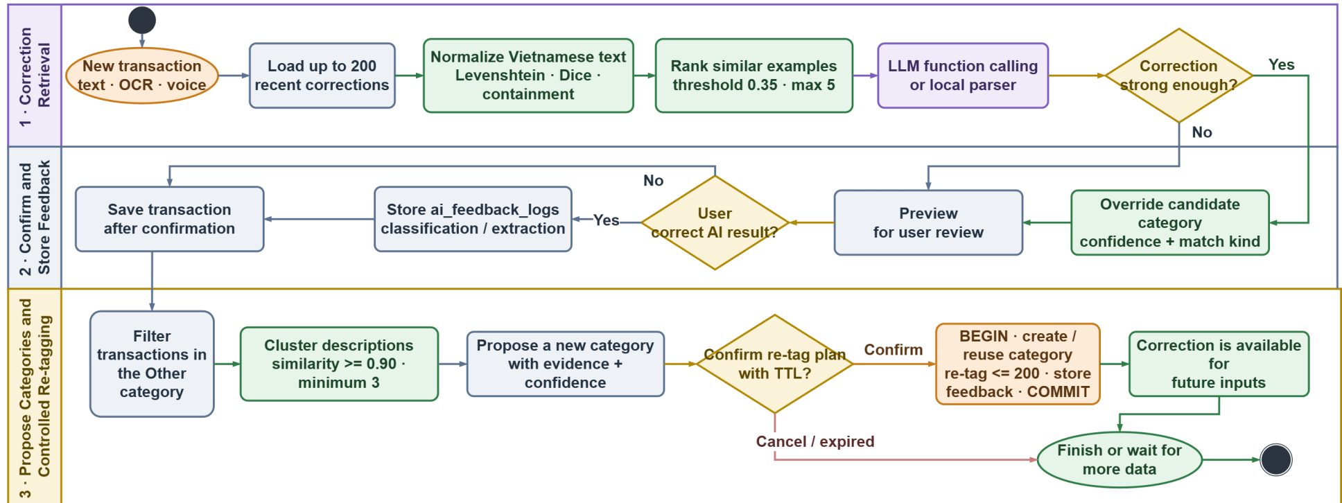
Hình 3.8: Luồng phân loại và correction retrieval; feedback chỉ được ghi sau khi người dùng xác nhận.
