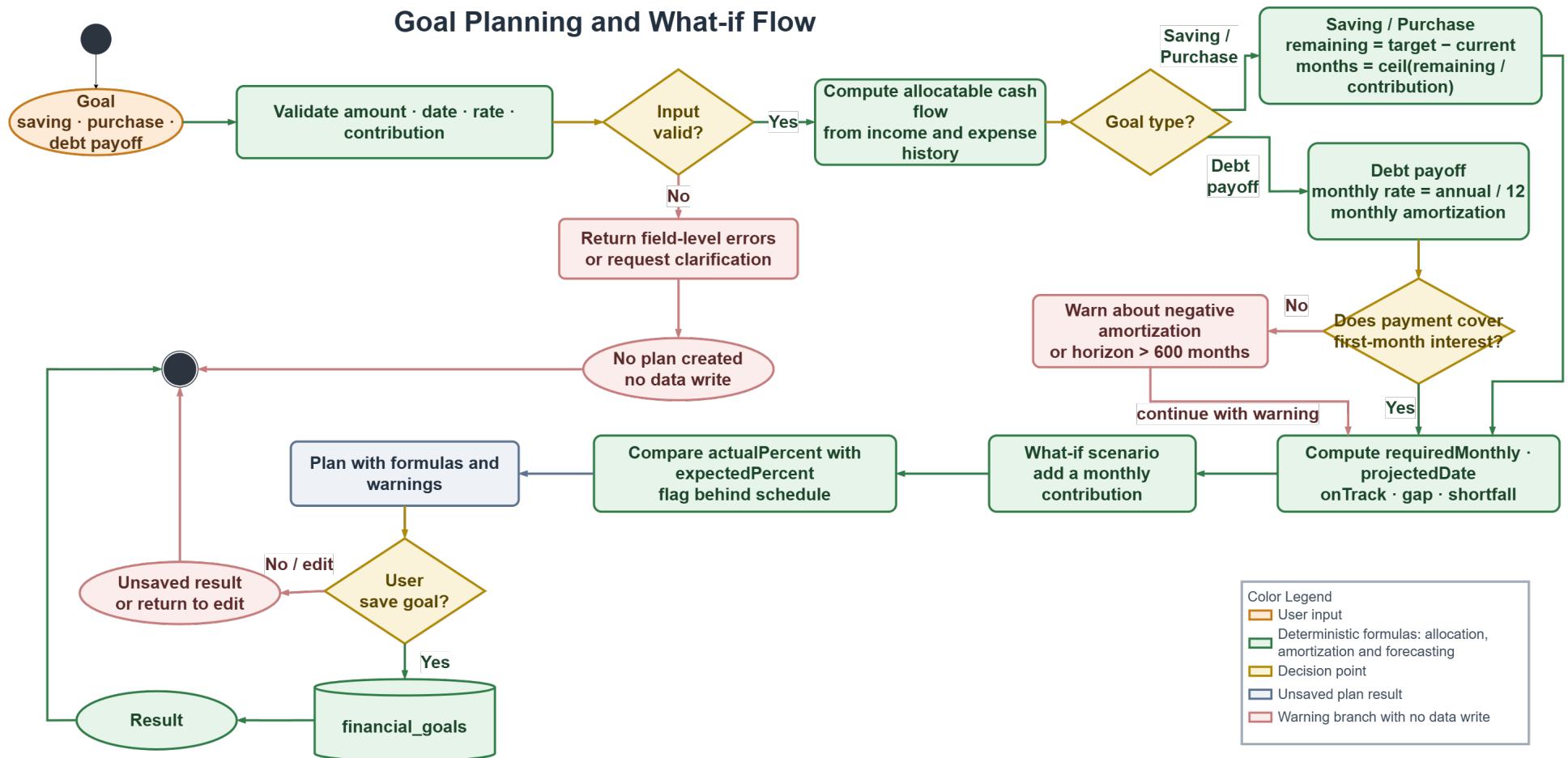
Hình 3.9: Flowchart lập kế hoạch mục tiêu và what-if; chỉ bước xác nhận cuối cùng mới lưu dữ liệu.
