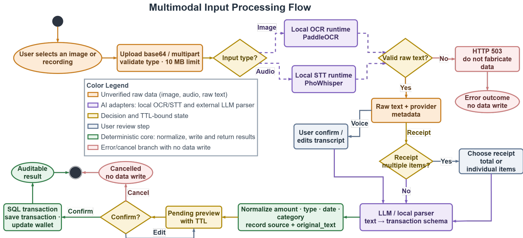
Hình 3.7: Flowchart xử lý ảnh và giọng nói; hai nhánh hội tụ vào pipeline văn bản sau khi raw text được kiểm tra.
