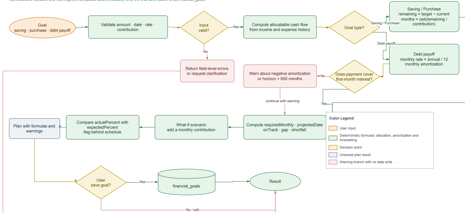
Hình 10: Flowchart lập kế hoạch mục tiêu và what-if; chỉ bước xác nhận cuối cùng mới lưu dữ liệu.
