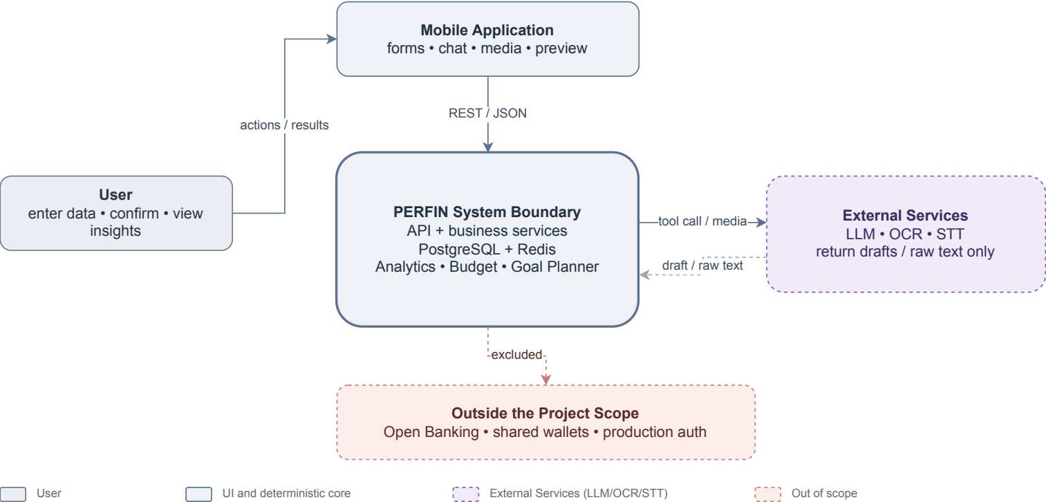
Hình 1: Ngữ cảnh và phạm vi của PERFIN; các dịch vụ LLM, OCR và STT nằm ngoài biên tin cậy dữ liệu.
