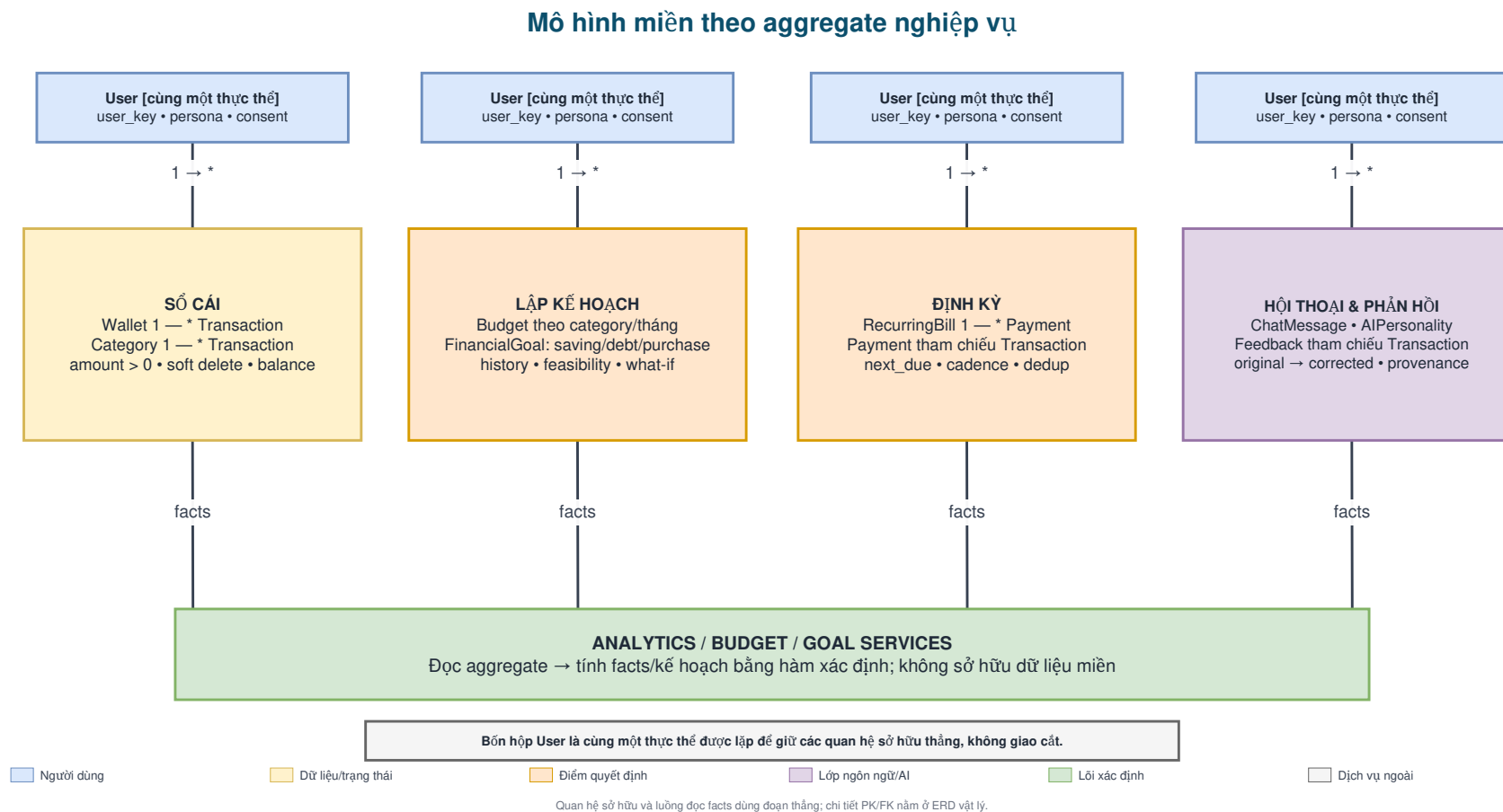
Hình 4: Mô hình miền theo aggregate nghiệp vụ. Các cụm dữ liệu tách khỏi service phân tích và lớp ngôn ngữ.
