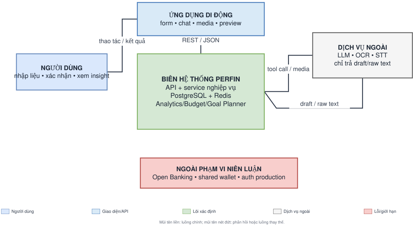
Hình 1: Sơ đồ ngữ cảnh và phạm vi hệ thống PERFIN. Người dùng tương tác với ứng dụng; các nhà cung cấp LLM, OCR và STT chỉ là dịch vụ hỗ trợ bên ngoài.
