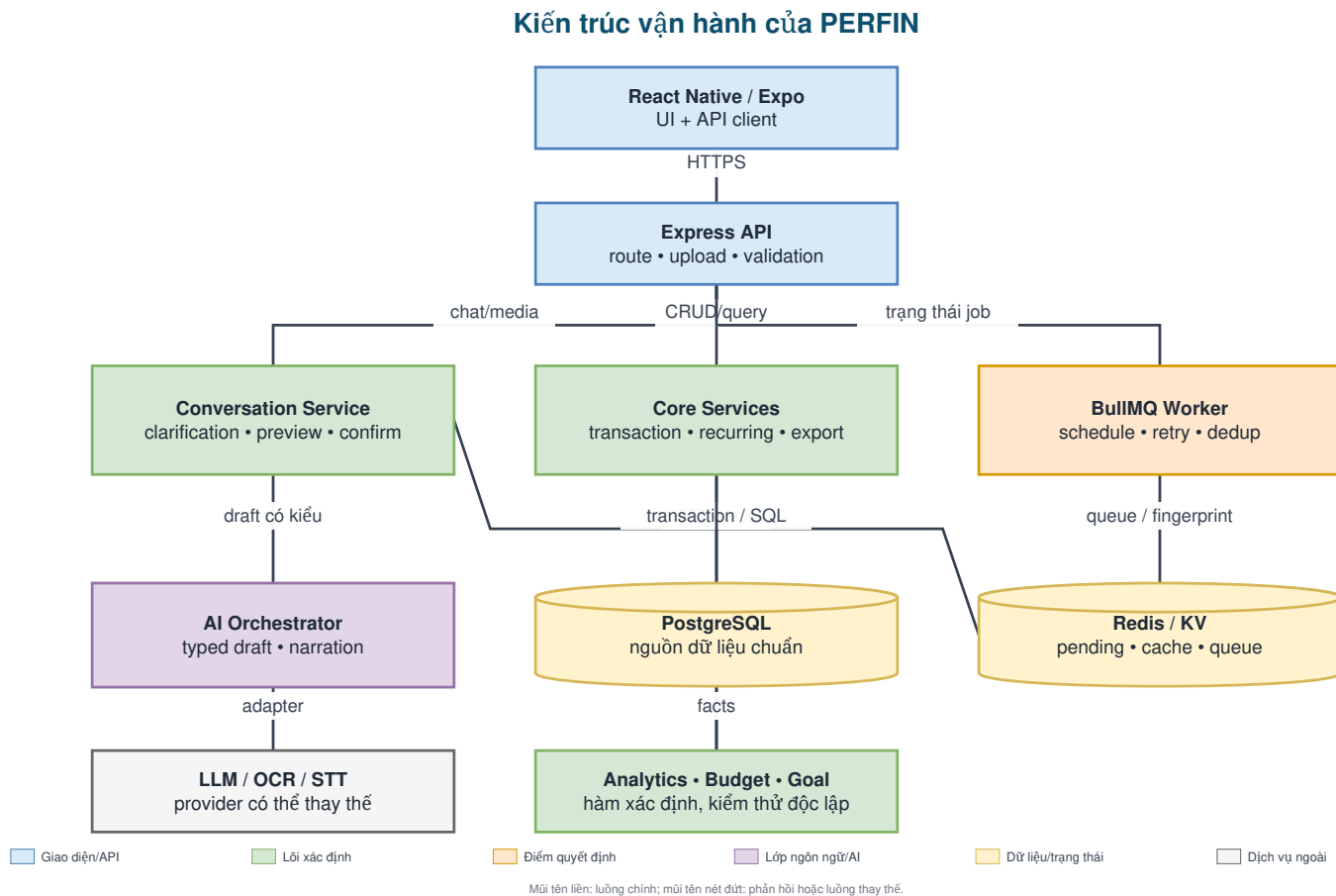
Hình 2: Kiến trúc vận hành của PERFIN. Logic xác định tạo và lưu facts; AI Orchestrator chỉ điều phối ngữ nghĩa.
