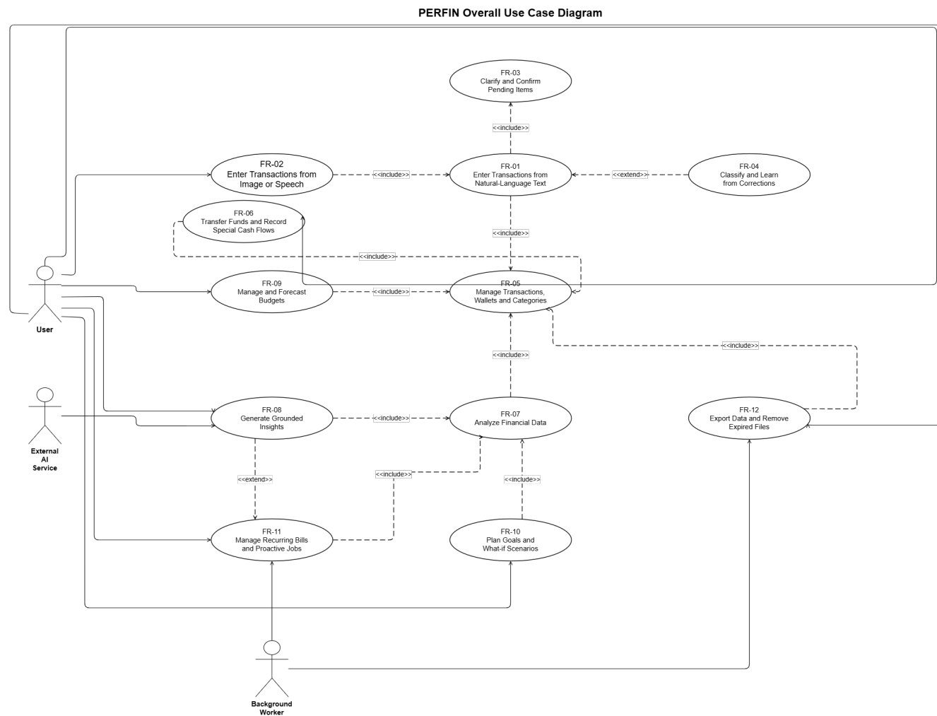
Hình 3.1: Sơ đồ use case tổng thể của PERFIN. Chi tiết từng chức năng được mô tả bằng bảng luồng thay cho mười hai sơ đồ riêng lẻ.
