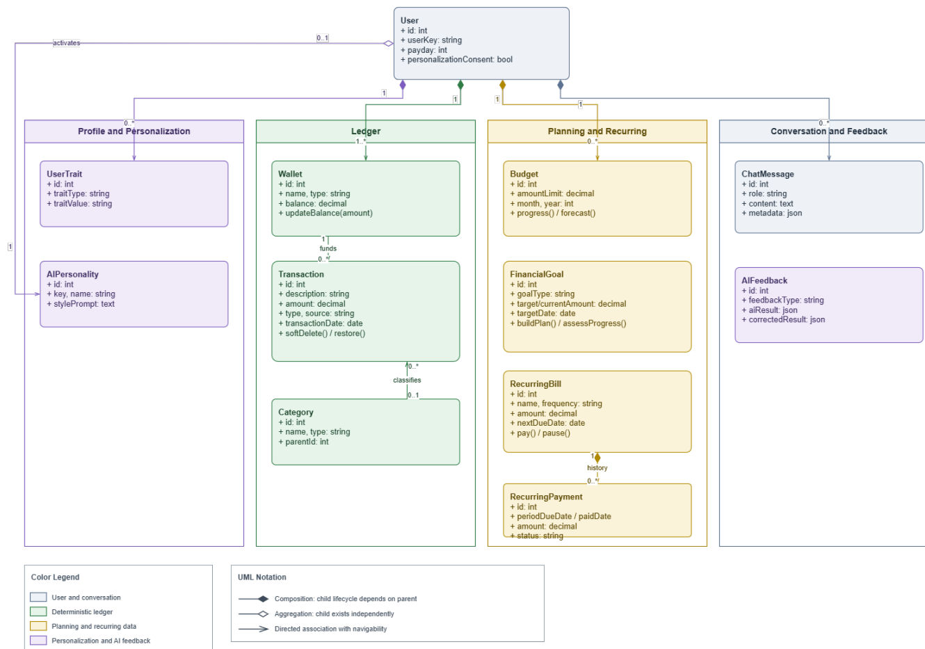
Hình 3.3: Class Diagram UML của miền PERFIN, tách sổ cái, kế hoạch, recurring và hội thoại/phản hồi.
