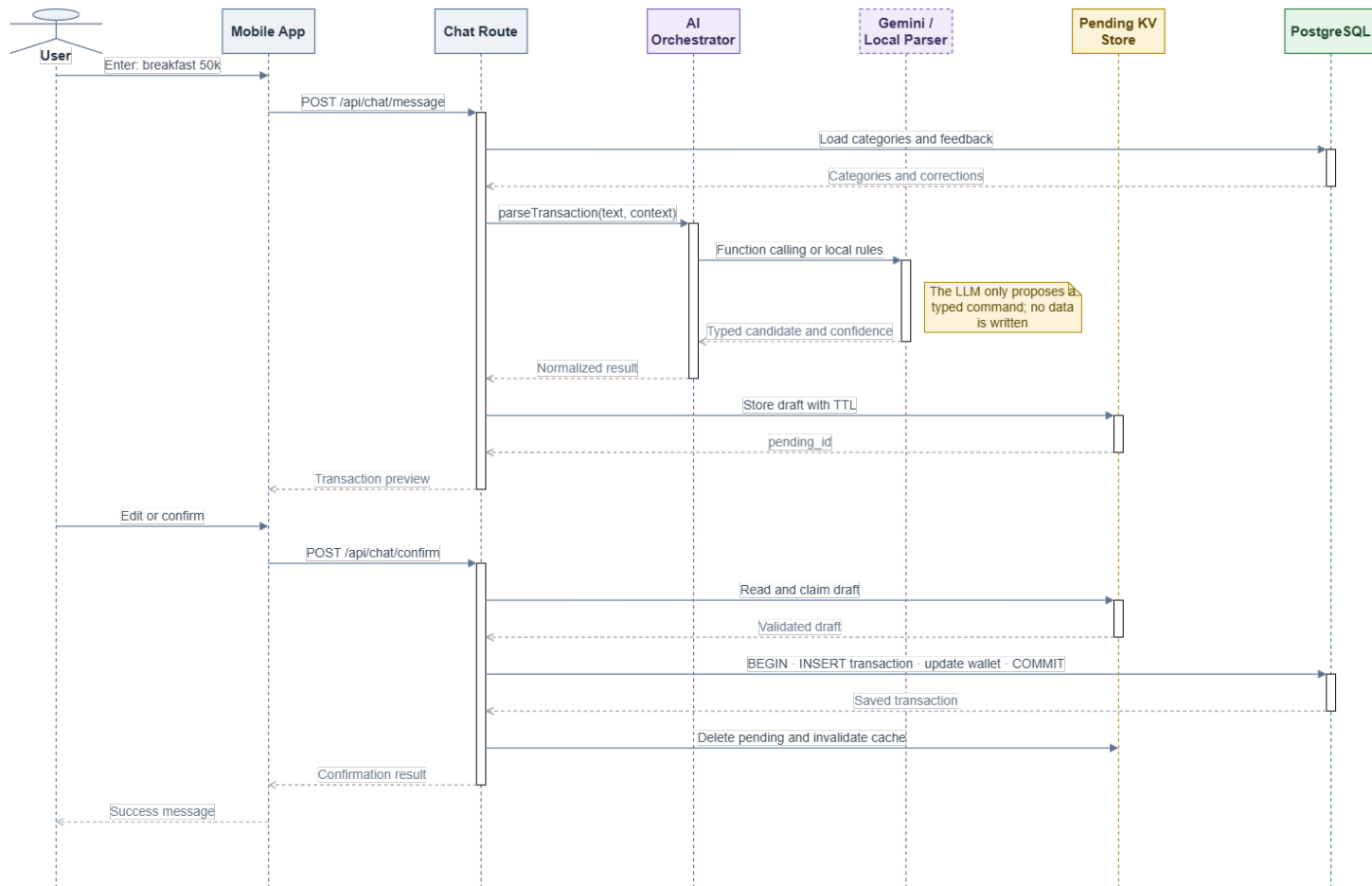
Hình 3.6: Sơ đồ tuần tự nhập giao dịch bằng văn bản; transaction ghi dữ liệu chỉ bắt đầu sau xác nhận.
