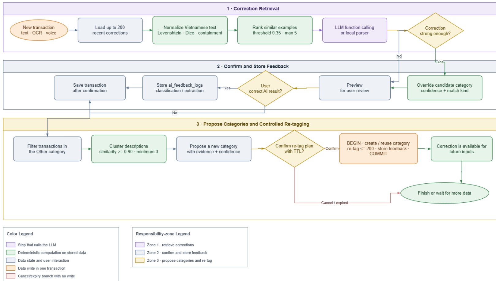
Hình 3.8: Luồng phân loại và correction retrieval; feedback chỉ được ghi sau khi người dùng xác nhận.
