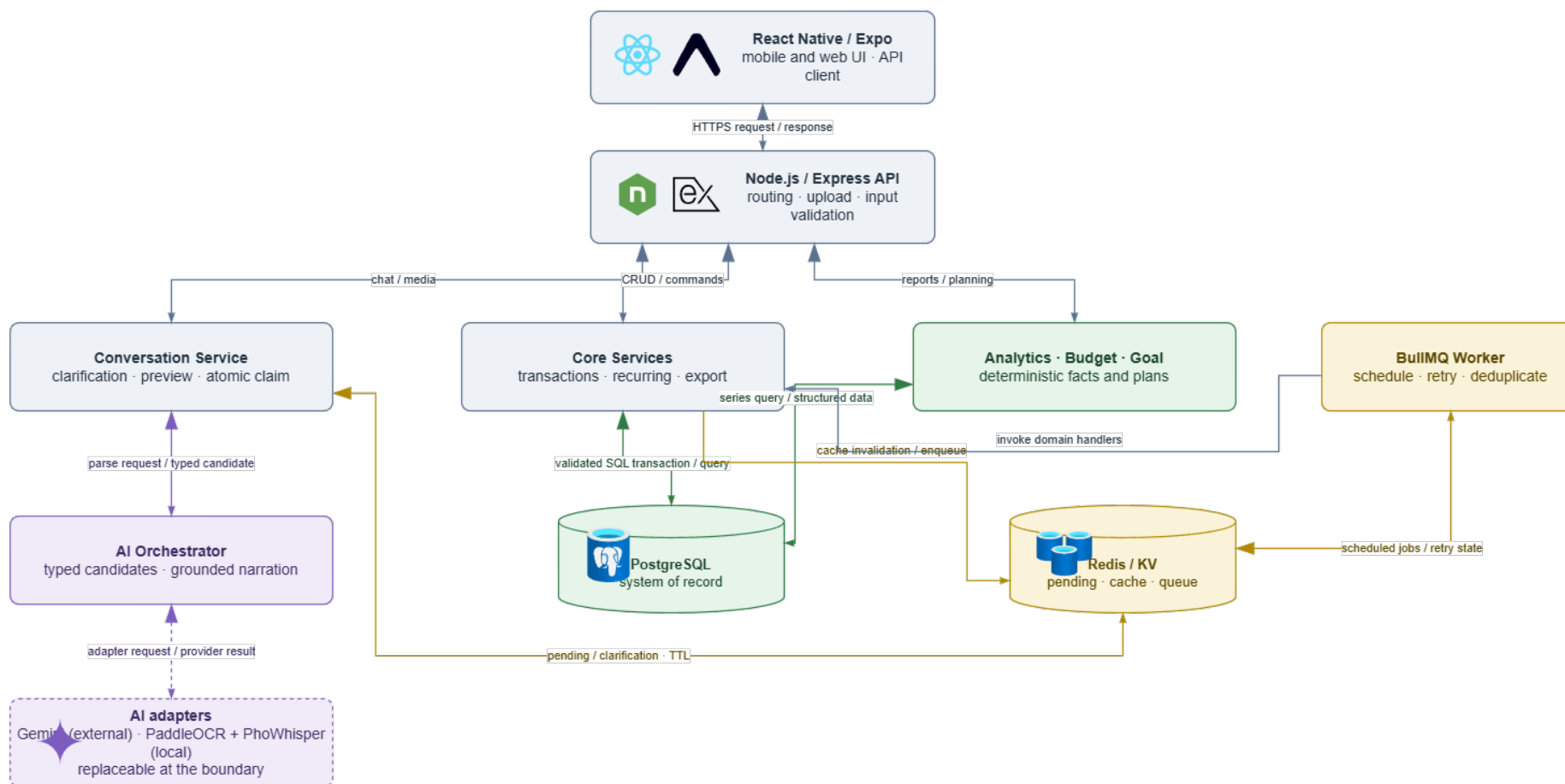
Hình 3.2: Kiến trúc vận hành của PERFIN; lõi xác định tạo và lưu facts, còn AI Orchestrator chỉ điều phối ngữ nghĩa.
