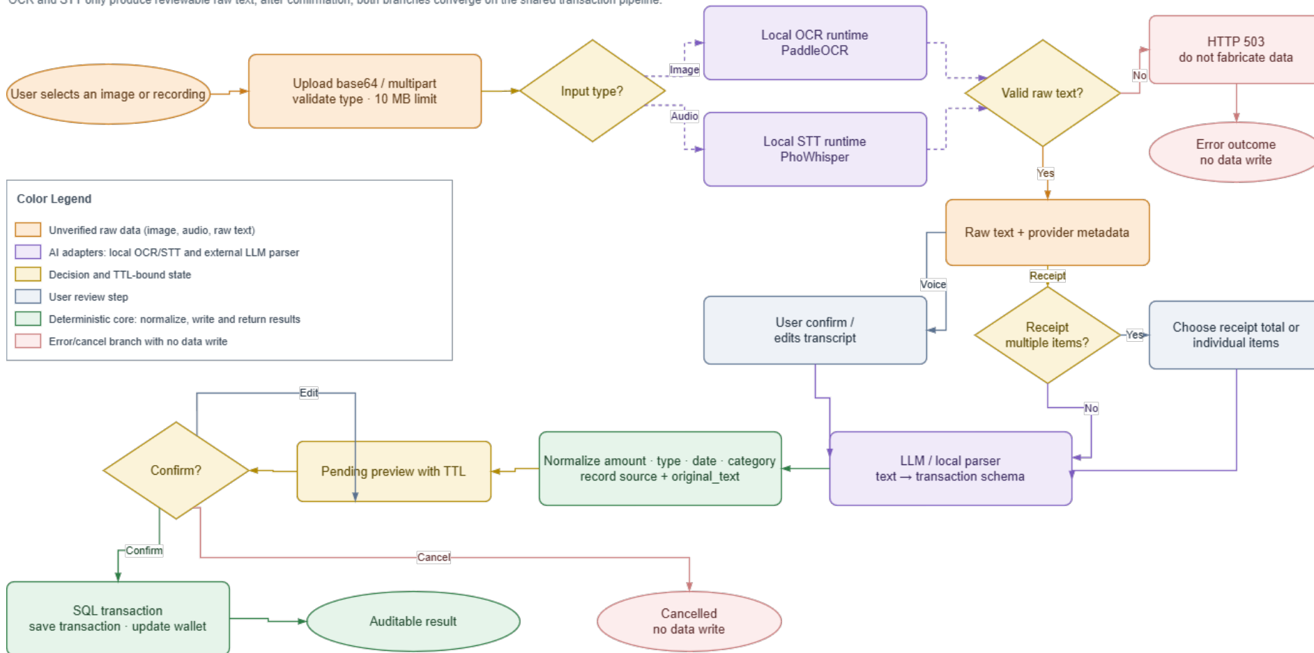
Hình 3.7: Flowchart xử lý ảnh và giọng nói; hai nhánh hội tụ vào pipeline văn bản sau khi raw text được kiểm tra.
