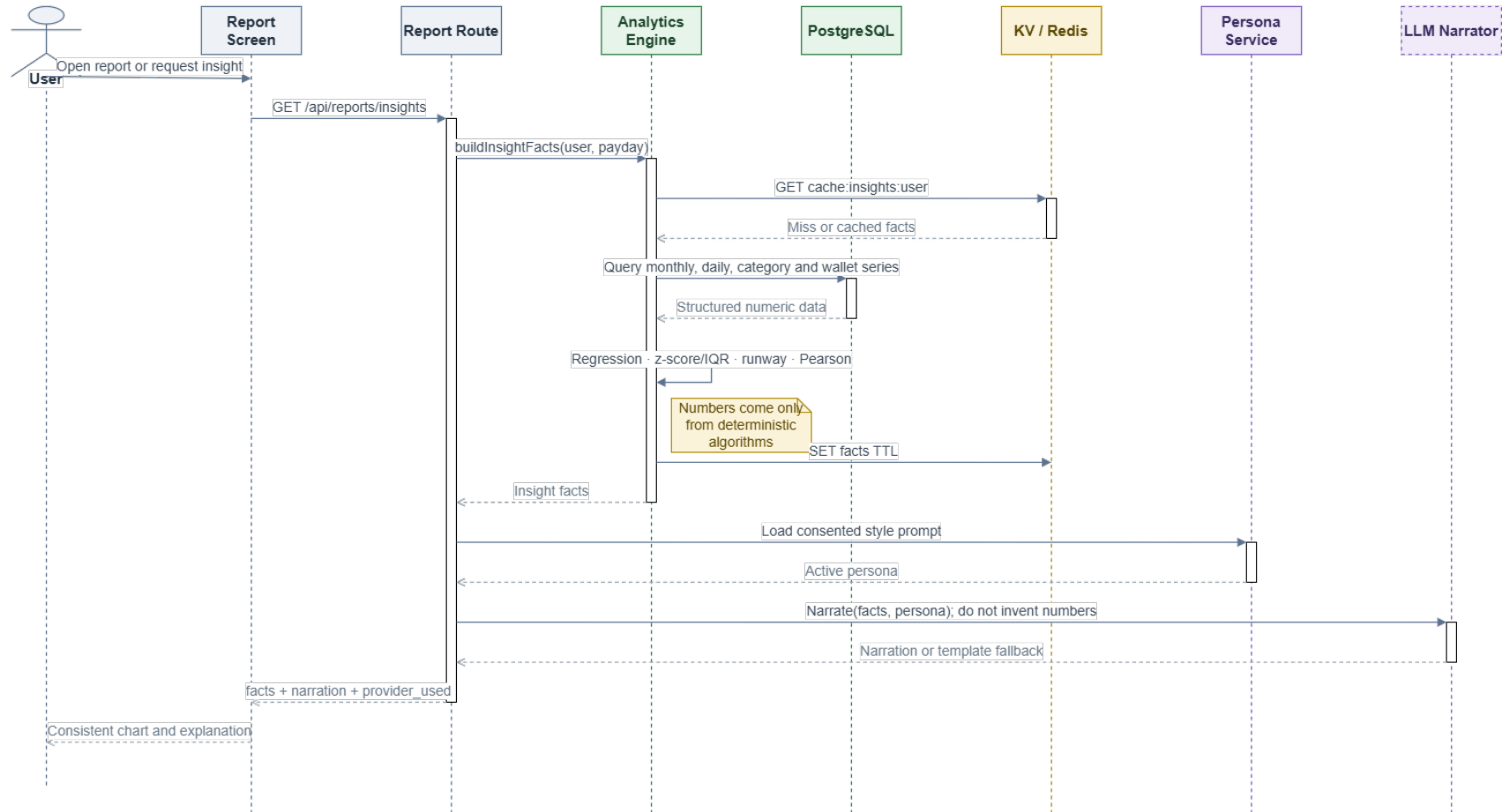
Hình 3.10: Sơ đồ tuần tự sinh insight; Analytics Engine trả facts trước khi persona/LLM diễn giải.
