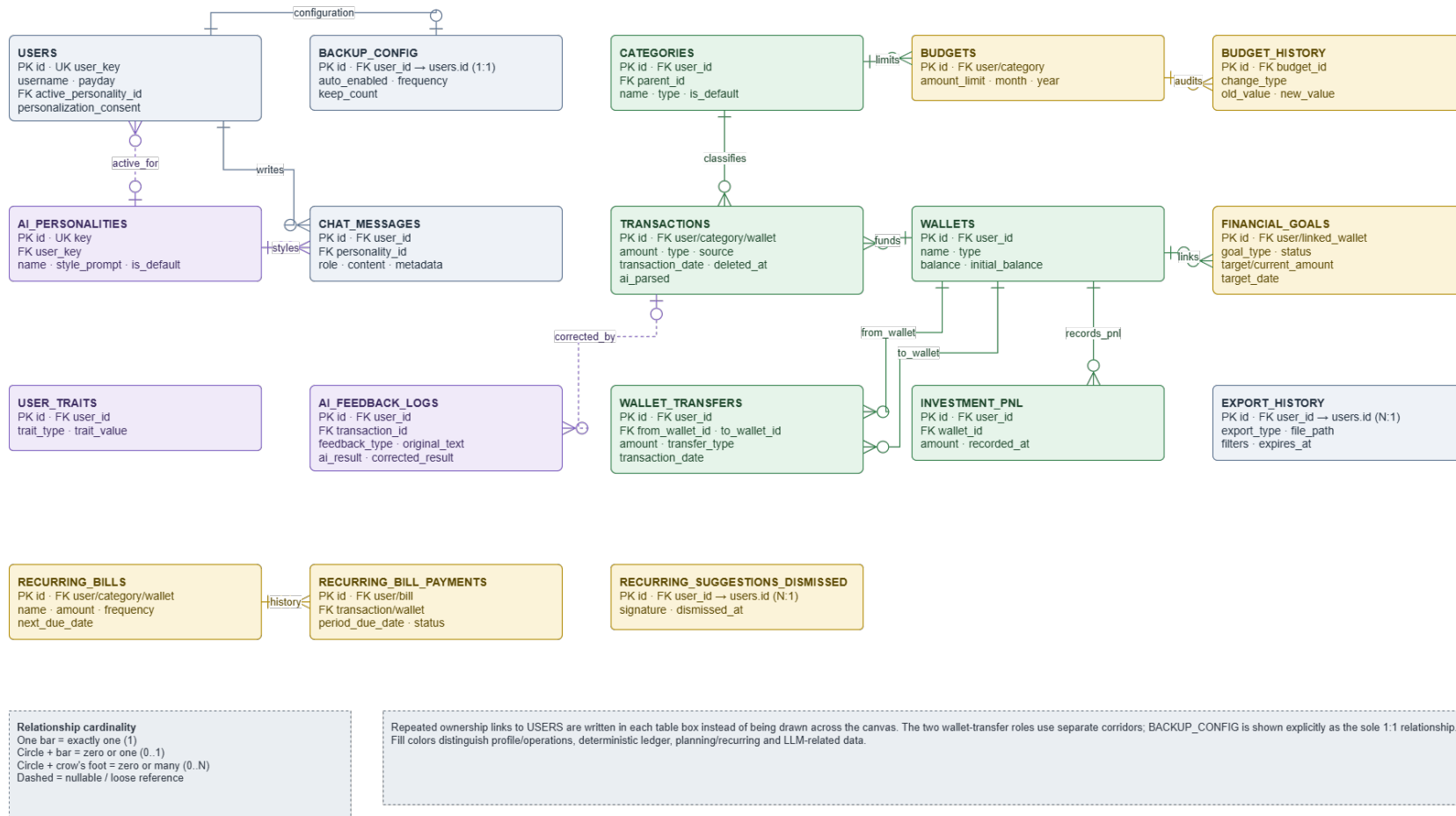
Hình 3.4: ERD vật lý được đối chiếu với chuỗi migration runtime; các khóa ngoại nghiệp vụ chính đi theo những hành lang trực giao tách biệt.
