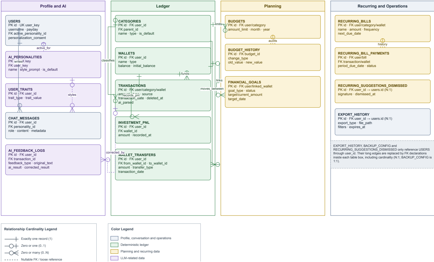
Hình 5: ERD vật lý được đối chiếu với chuỗi migration runtime; các khóa ngoại nghiệp vụ chính được thể hiện bằng quan hệ thẳng.
