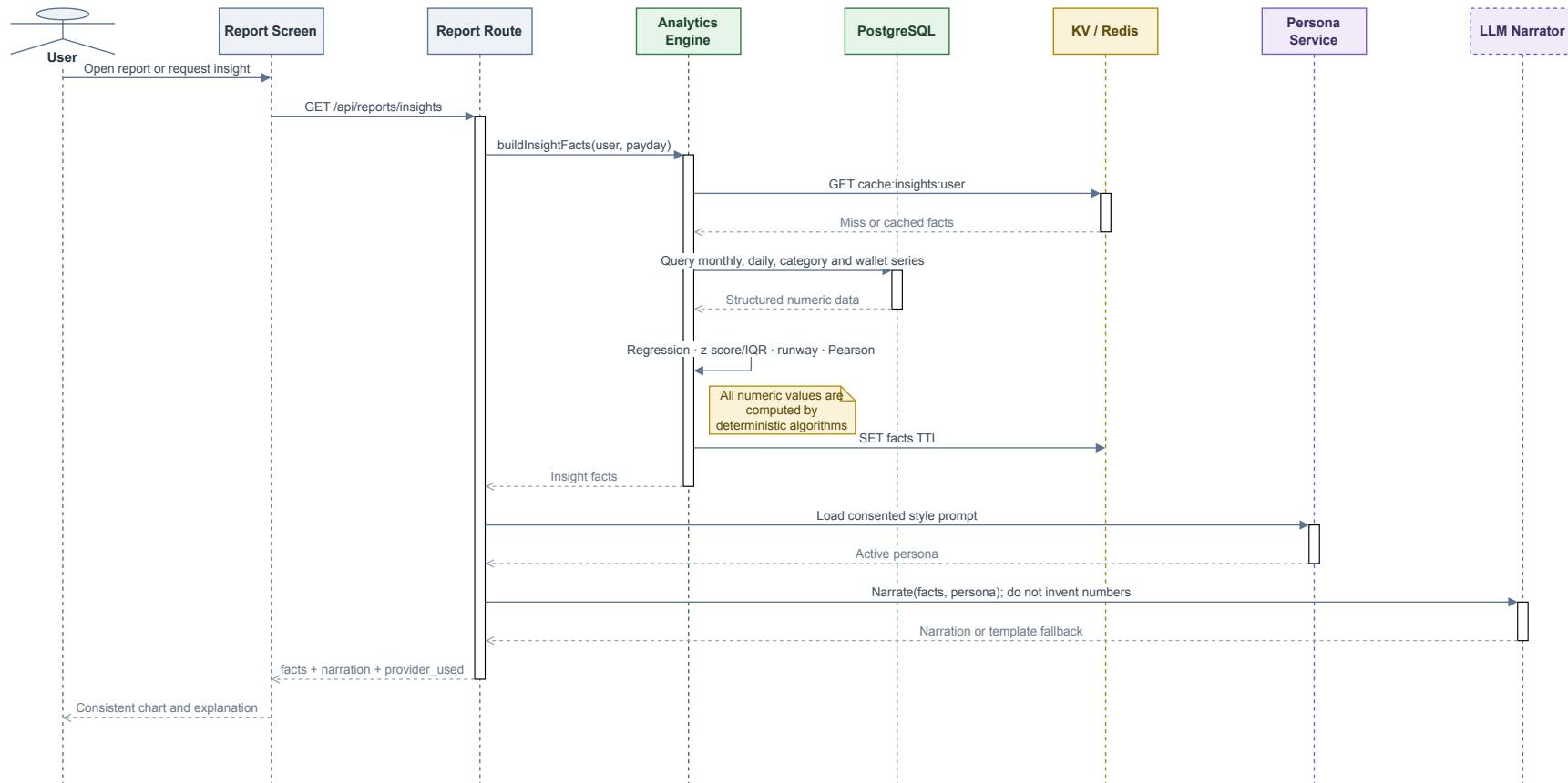
Hình 11: Sơ đồ tuần tự sinh insight; Analytics Engine trả facts trước khi persona/LLM diễn giải.
