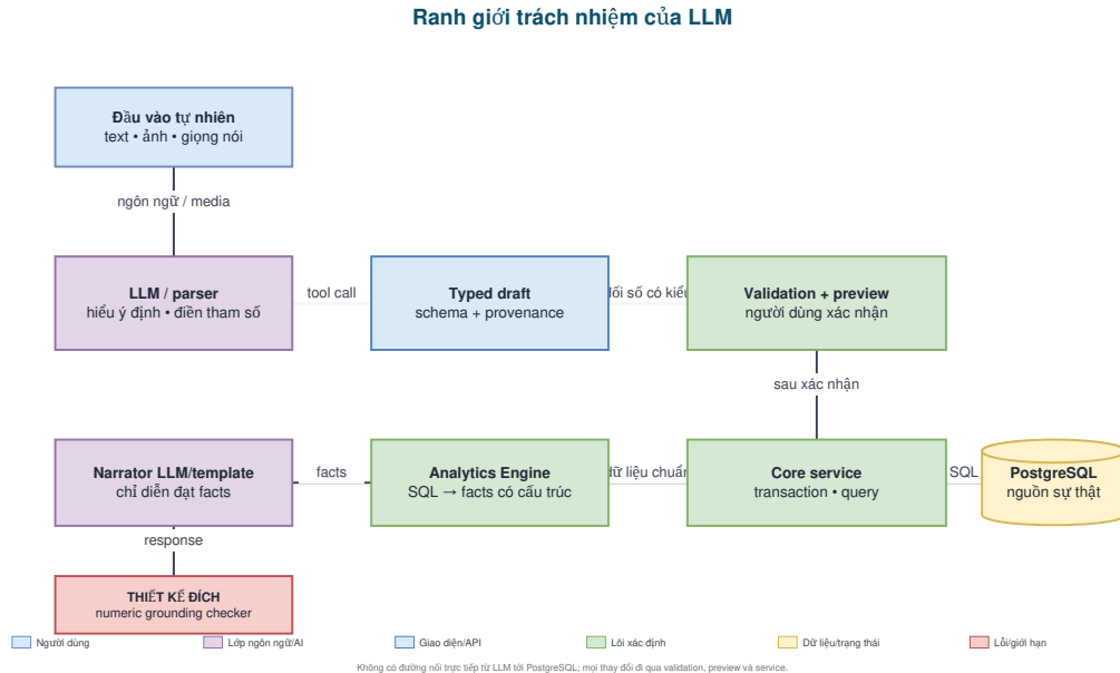
Hình 6: Ranh giới trách nhiệm của LLM: dữ liệu và facts được tạo ở lỗi xác định; LLM chỉ chuyển đổi ngữ nghĩa và diễn giải.
