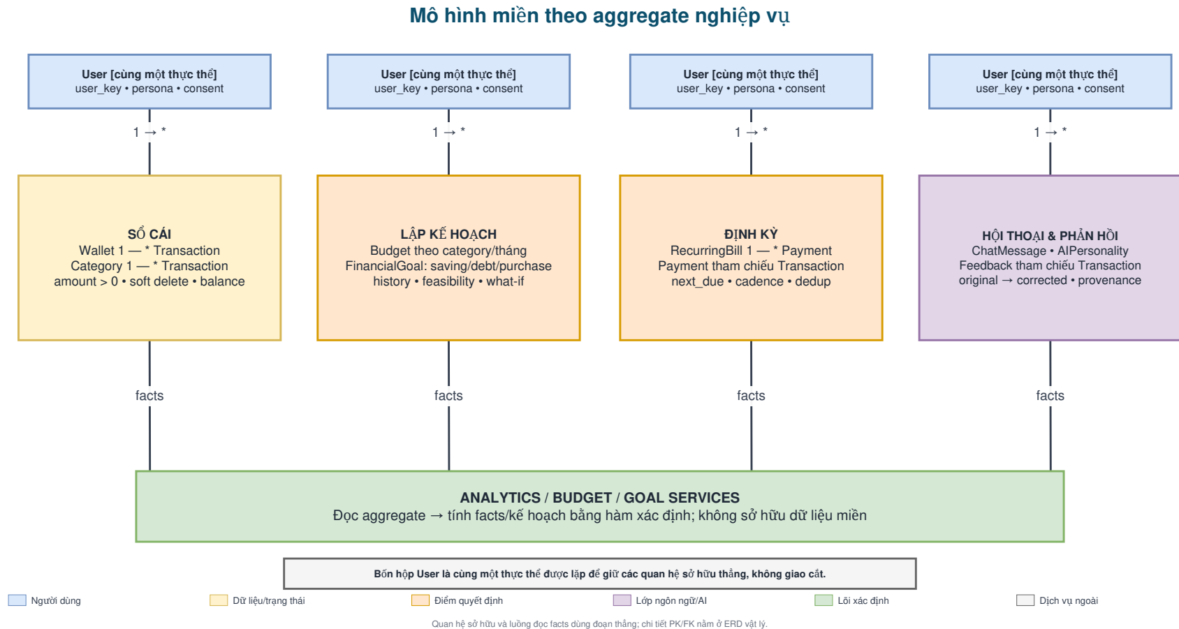
Hình 4: Mô hình miền theo aggregate nghiệp vụ. Các cụm dữ liệu tách khỏi service phân tích và lớp ngôn ngữ.
