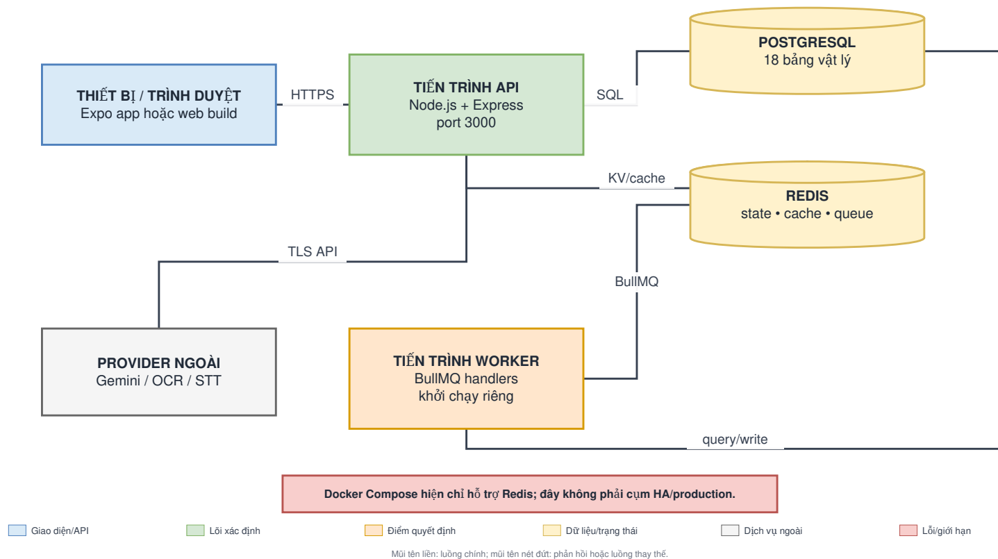
Hình 3: Sơ đồ triển khai nguyên mẫu. Frontend, API, worker, PostgreSQL và Redis thuộc môi trường demo; provider AI được gọi qua mạng.
