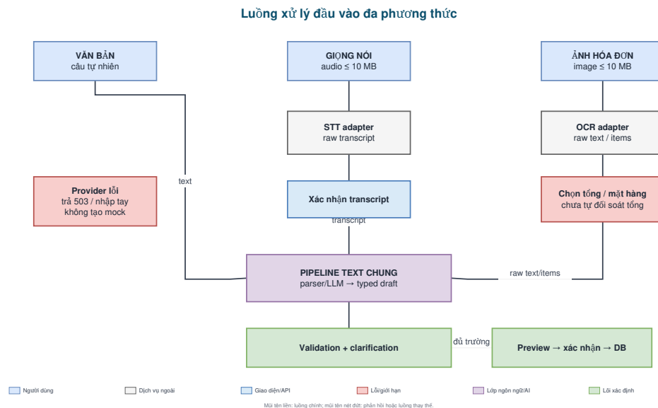
Hình 9: Luồng xử lý đầu vào đa phương thức. Voice và ảnh hội tụ vào pipeline text chung sau bước xác nhận.
