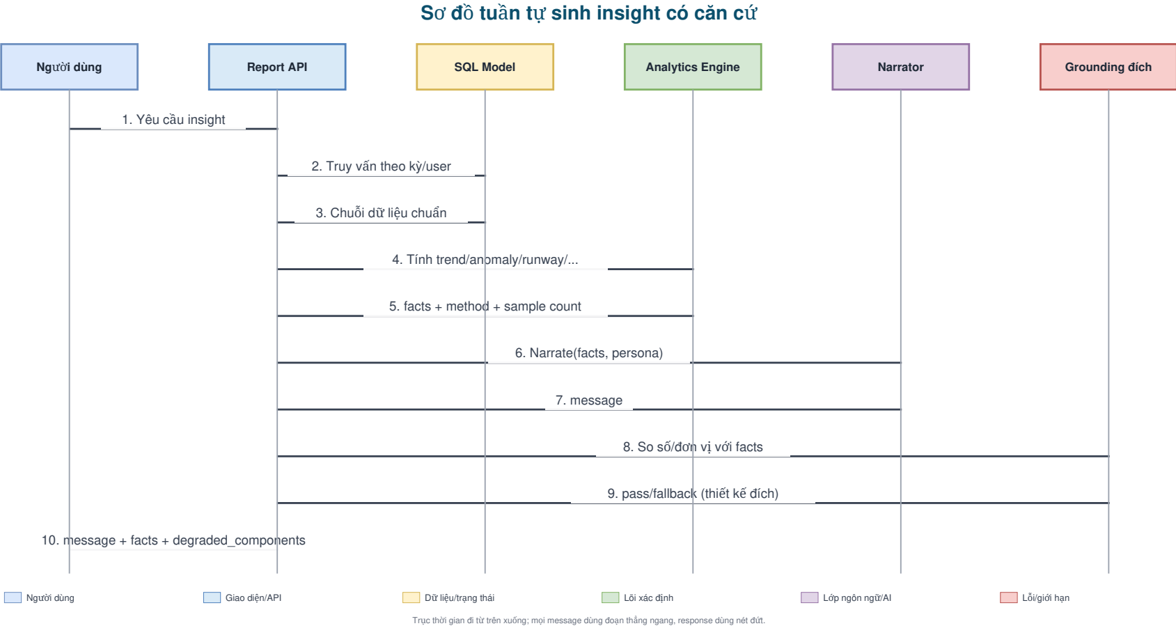
Hình 11: Sơ đồ tuần tự sinh insight có căn cứ. Response trả cả thông điệp và facts để truy vết.
