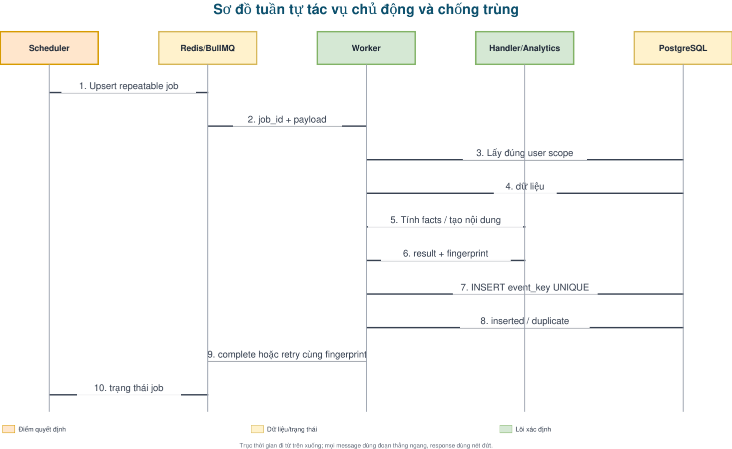
Hình 13: Sơ đồ tuần tự tác vụ chủ động và cơ chế chống hiệu ứng lặp khi retry.
