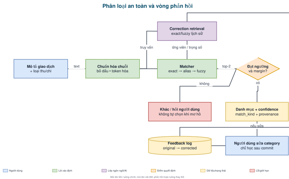
Hình 10: Luồng phản hồi và cá nhân hóa phân loại bằng correction retrieval, không phải fine-tuning.
