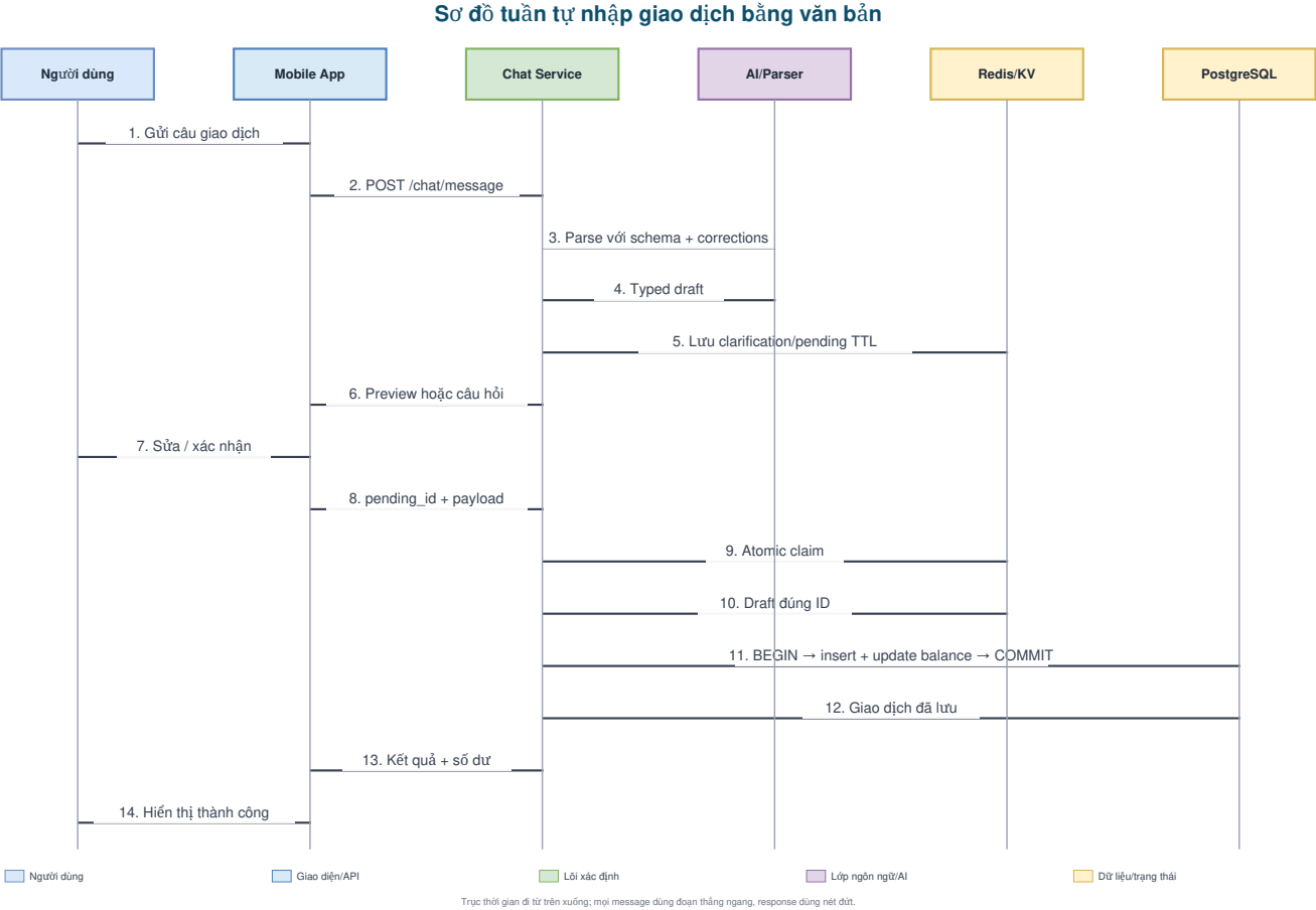
Hình 8: Sơ đồ tuần tự nhập giao dịch bằng văn bản. LLM nằm ngoài transaction ghi dữ liệu.
