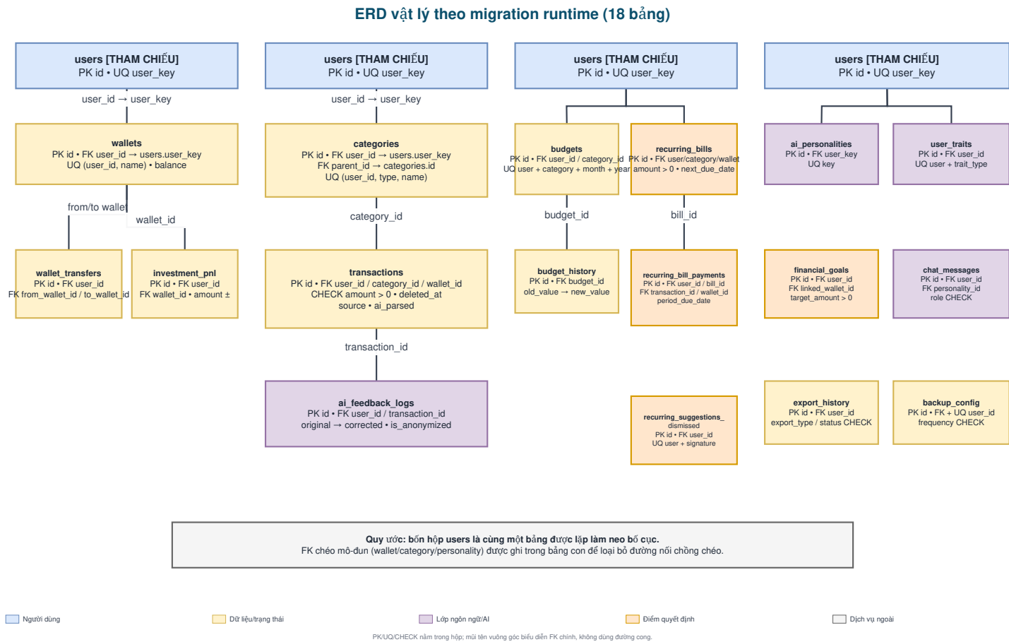
Hình 5: Sơ đồ quan hệ thực thể vật lý được đối chiếu với chuỗi migration runtime.
