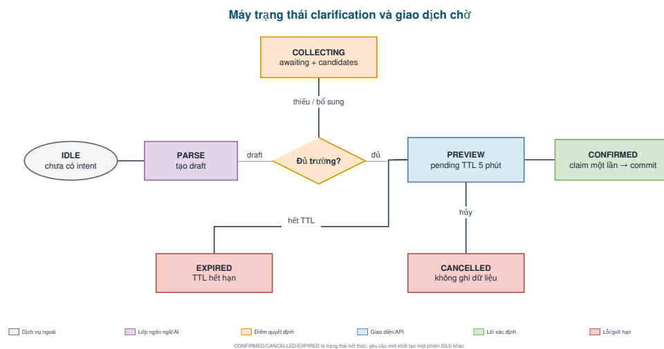
Hình 7: Máy trạng thái hội thoại và giao dịch chờ xác nhận.
