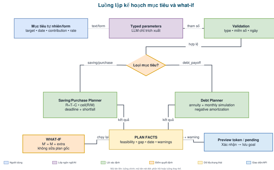
Hình 12: Luồng lập kế hoạch mục tiêu và mô phỏng what-if.
