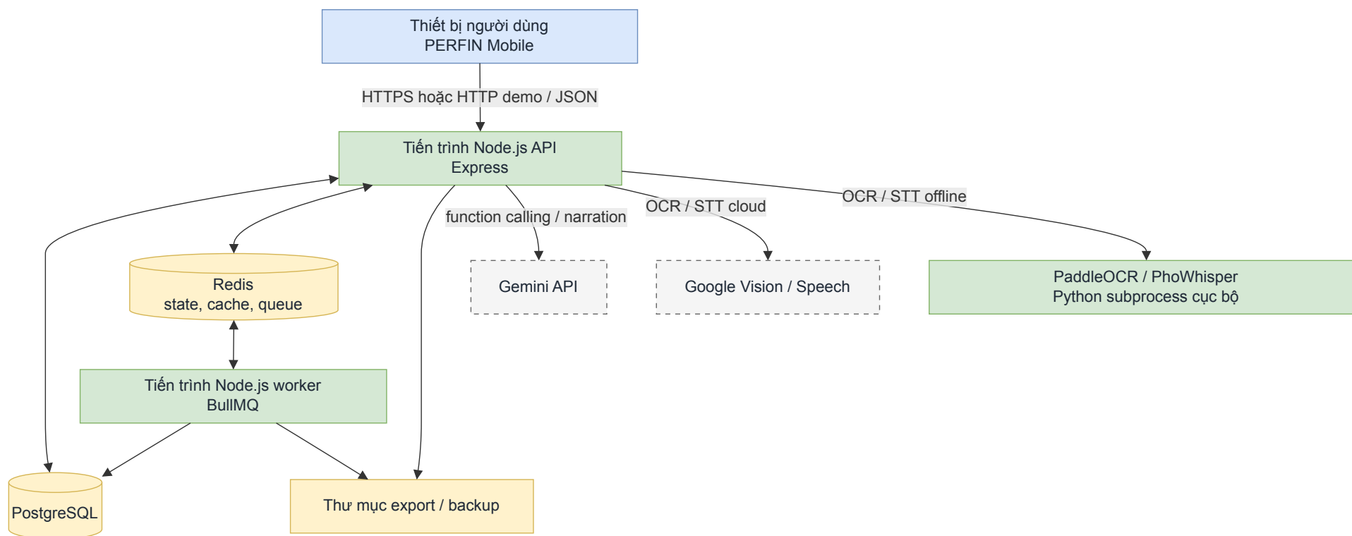
Hình 3: Sơ đồ triển khai nguyên mẫu. Frontend, API, worker, PostgreSQL và Redis thuộc môi trường demo; provider AI được gọi qua mạng.
