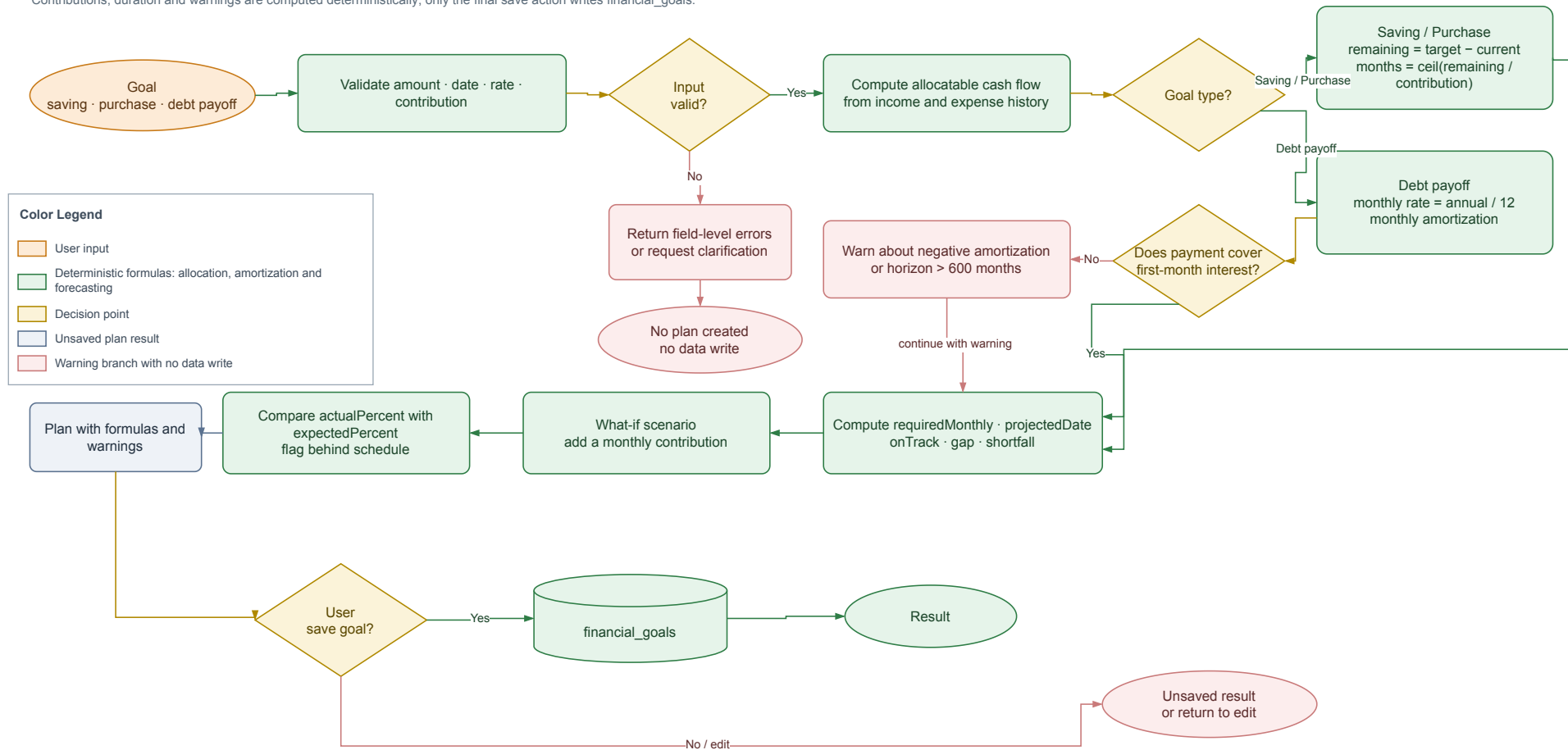
Hình 3.11: Flowchart lập kế hoạch mục tiêu và what-if; chỉ bước xác nhận cuối cùng mới lưu dữ liệu.
