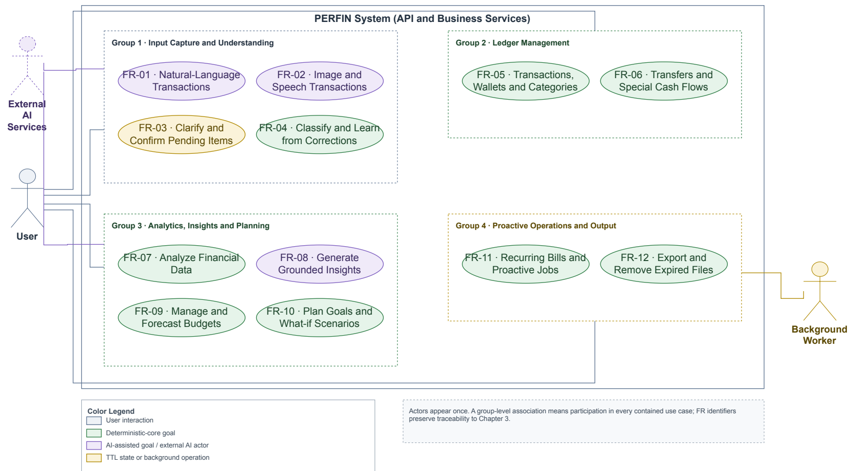
Hình 3.1: Sơ đồ use case tổng thể của PERFIN. Chi tiết từng chức năng được mô tả bằng bảng luồng thay cho mười hai sơ đồ riêng lẻ.
