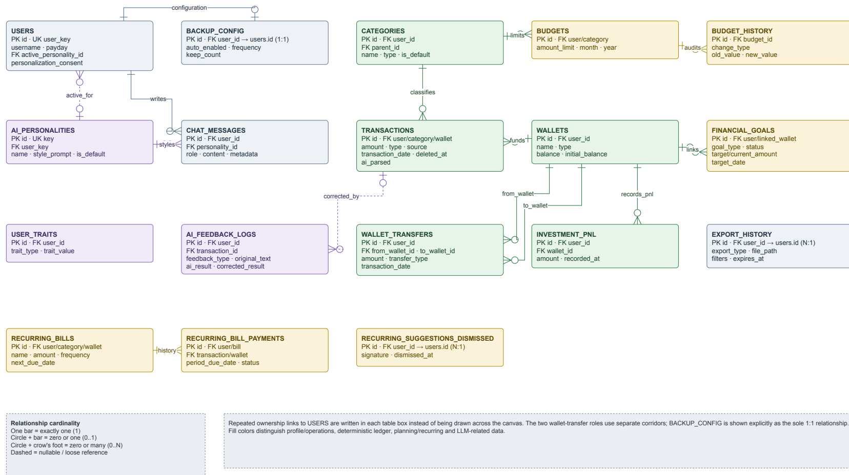
Hình 3.6: ERD vật lý được đối chiếu với chuỗi migration runtime; các khóa ngoại nghiệp vụ chính đi theo những hành lang trực giao tách biệt.
