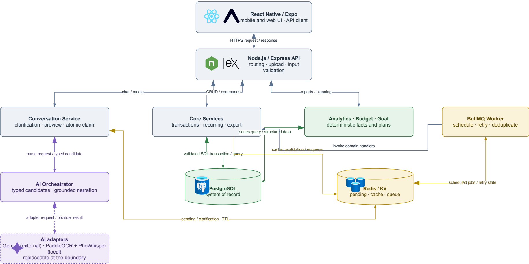
Hình 3.4: Kiến trúc vận hành của PERFIN; lõi xác định tạo và lưu facts, còn AI Orchestrator chỉ điều phối ngữ nghĩa.
