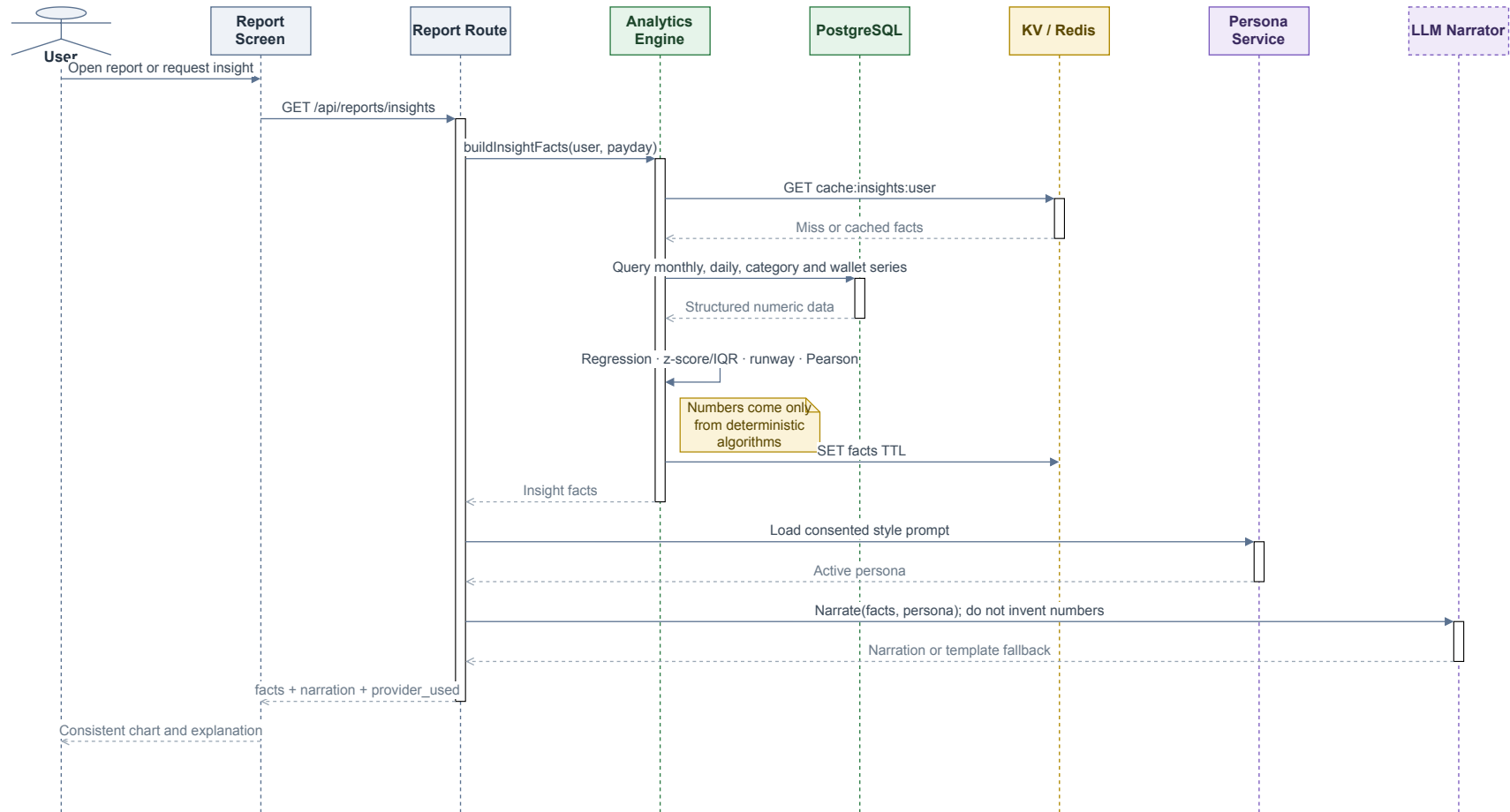
Hình 3.12: Sơ đồ tuần tự sinh insight; Analytics Engine trả facts trước khi persona/LLM diễn giải.
