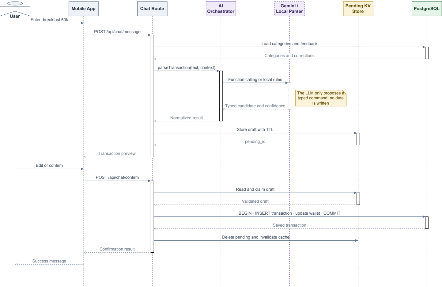
Hình 3.8: Sơ đồ tuần tự nhập giao dịch bằng văn bản; transaction ghi dữ liệu chỉ bắt đầu sau xác nhận.
