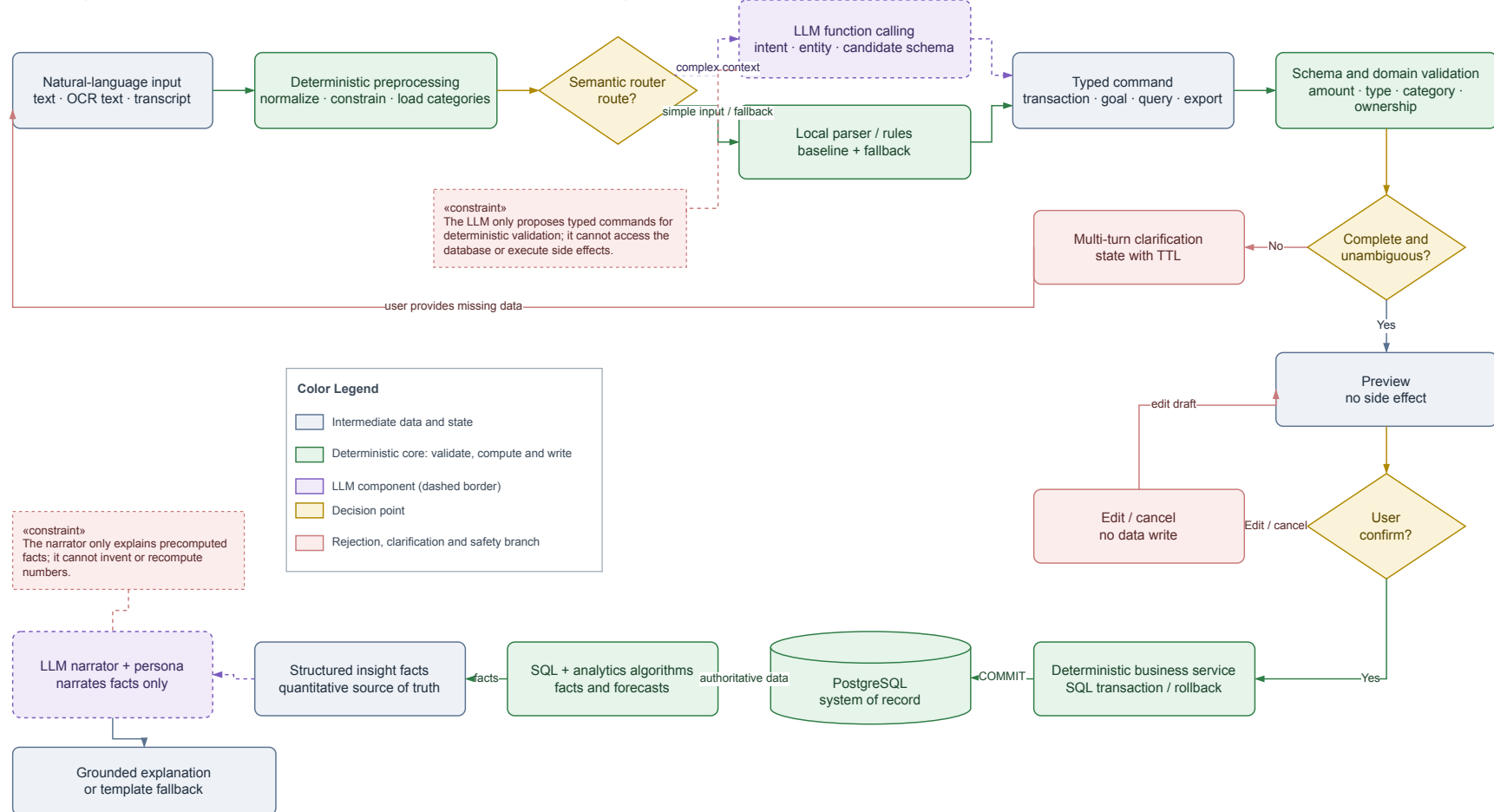
Hình 3.7: Ranh giới trách nhiệm của LLM: typed draft và narration nằm ngoài lõi validation, tính toán và ghi dữ liệu.
