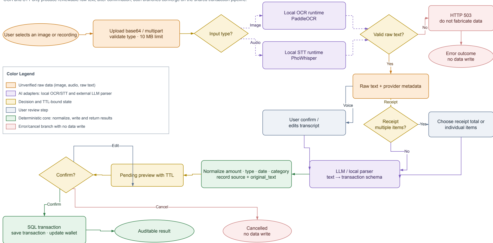
Hình 3.9: Flowchart xử lý ảnh và giọng nói; hai nhánh hội tụ vào pipeline văn bản sau khi raw text được kiểm tra.
