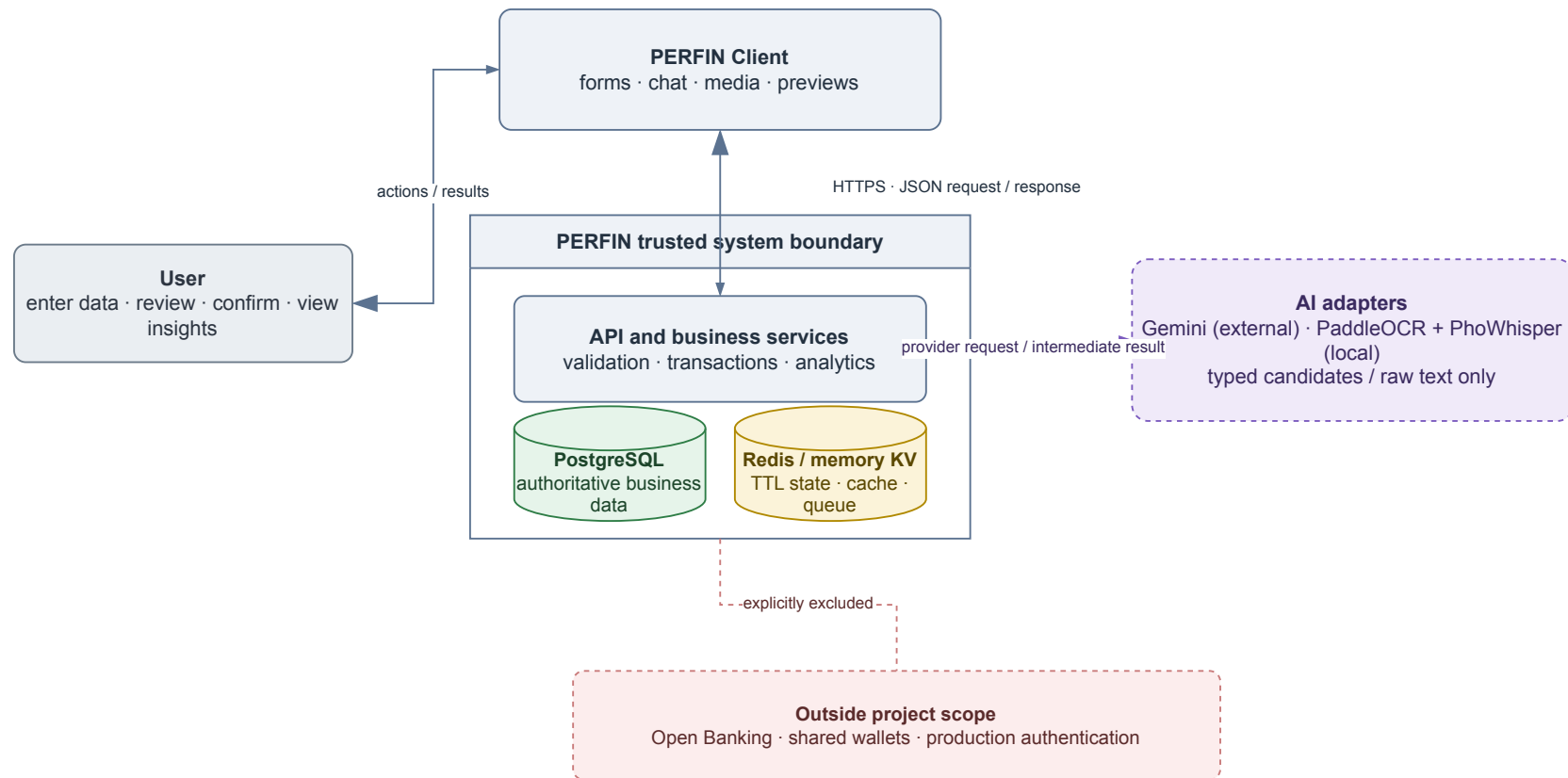
Hình 1.1: Ngữ cảnh và phạm vi của PERFIN; các dịch vụ LLM, OCR và STT nằm ngoài biên tin cậy dữ liệu.
