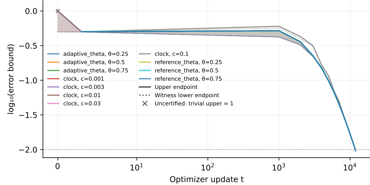
Frozen retrieval · ADAM
