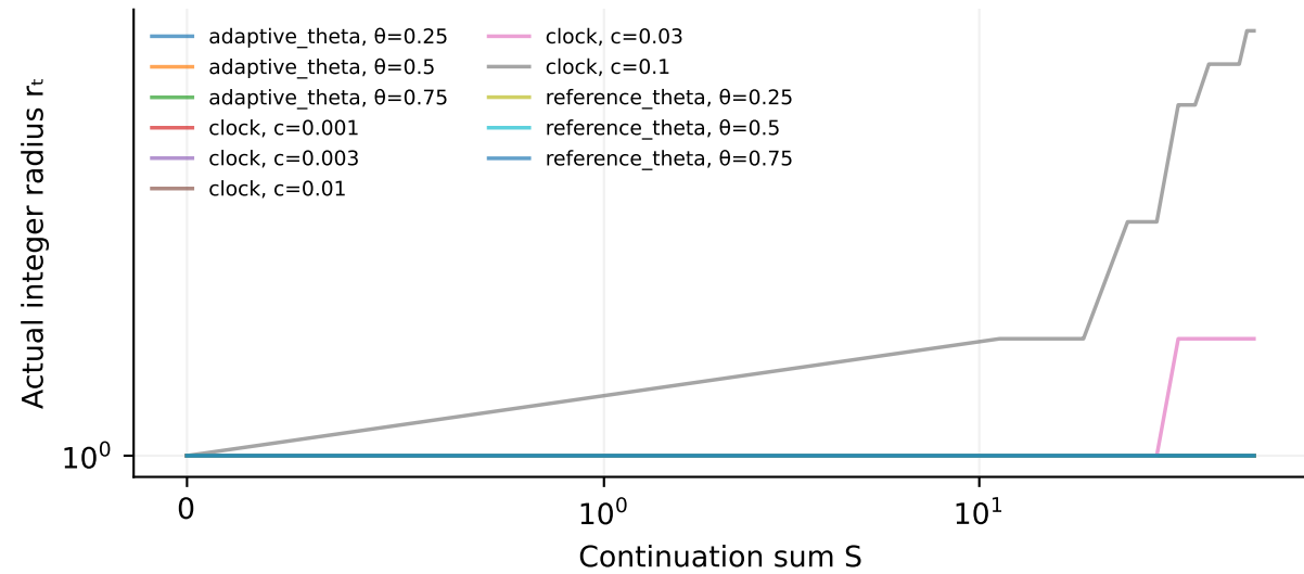
Frozen retrieval · SGD — actual probe radius
