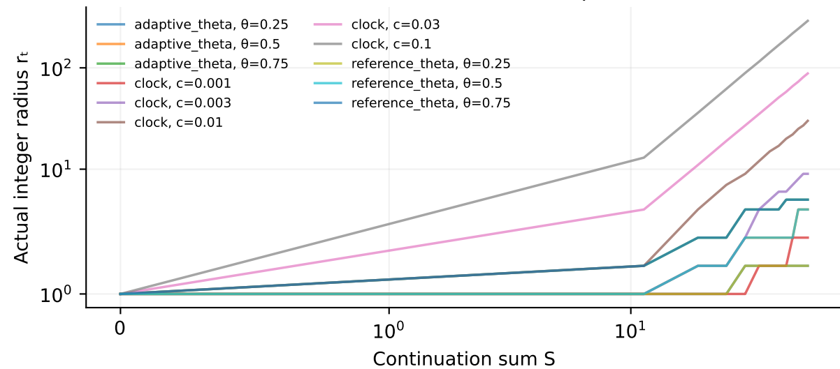
Frozen retrieval · ADAM — actual probe radius
