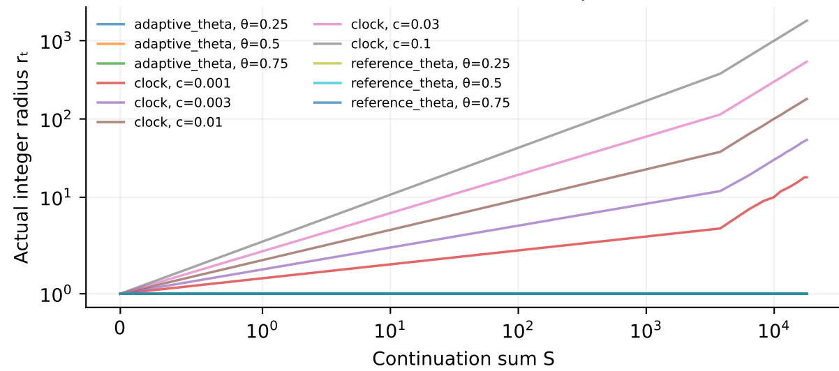
Learned retrieval · ADAM — actual probe radius
