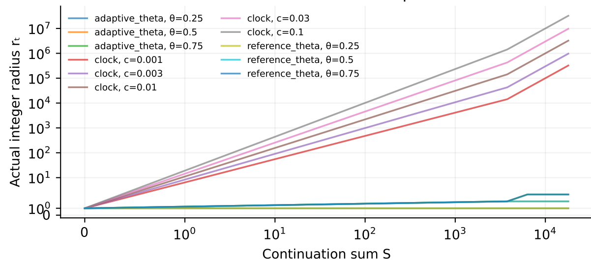
Frozen retrieval · ADAM — actual probe radius
