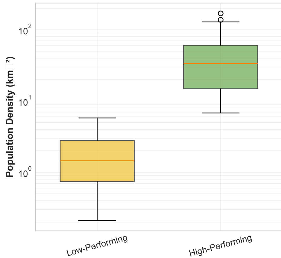
Population Density
