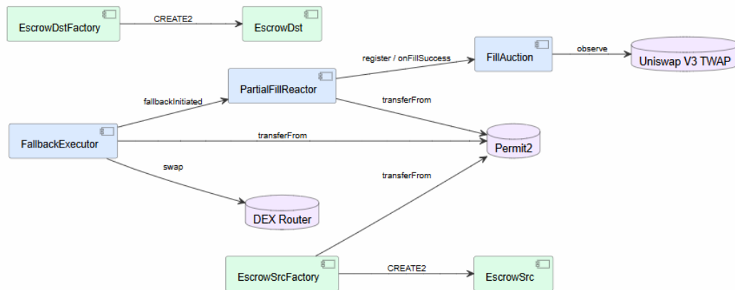
Hình 3.3: Sơ đồ phụ thuộc giữa các hợp đồng.
