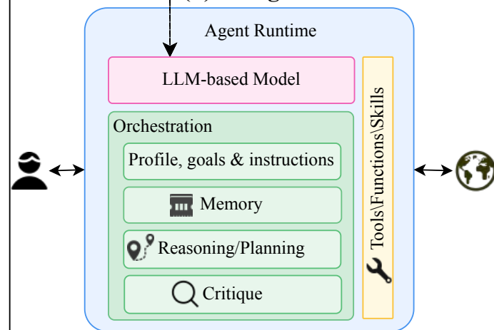
(d) AI Agent
