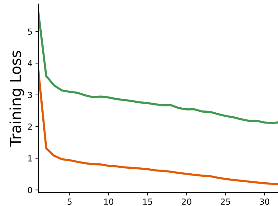
LAION-400M
