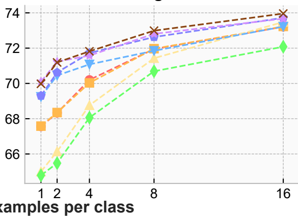
ImageNet
