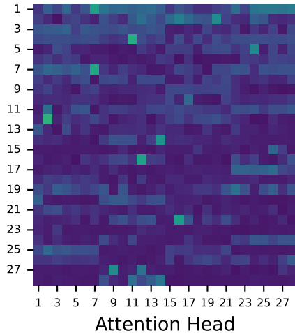
Wikitext2
