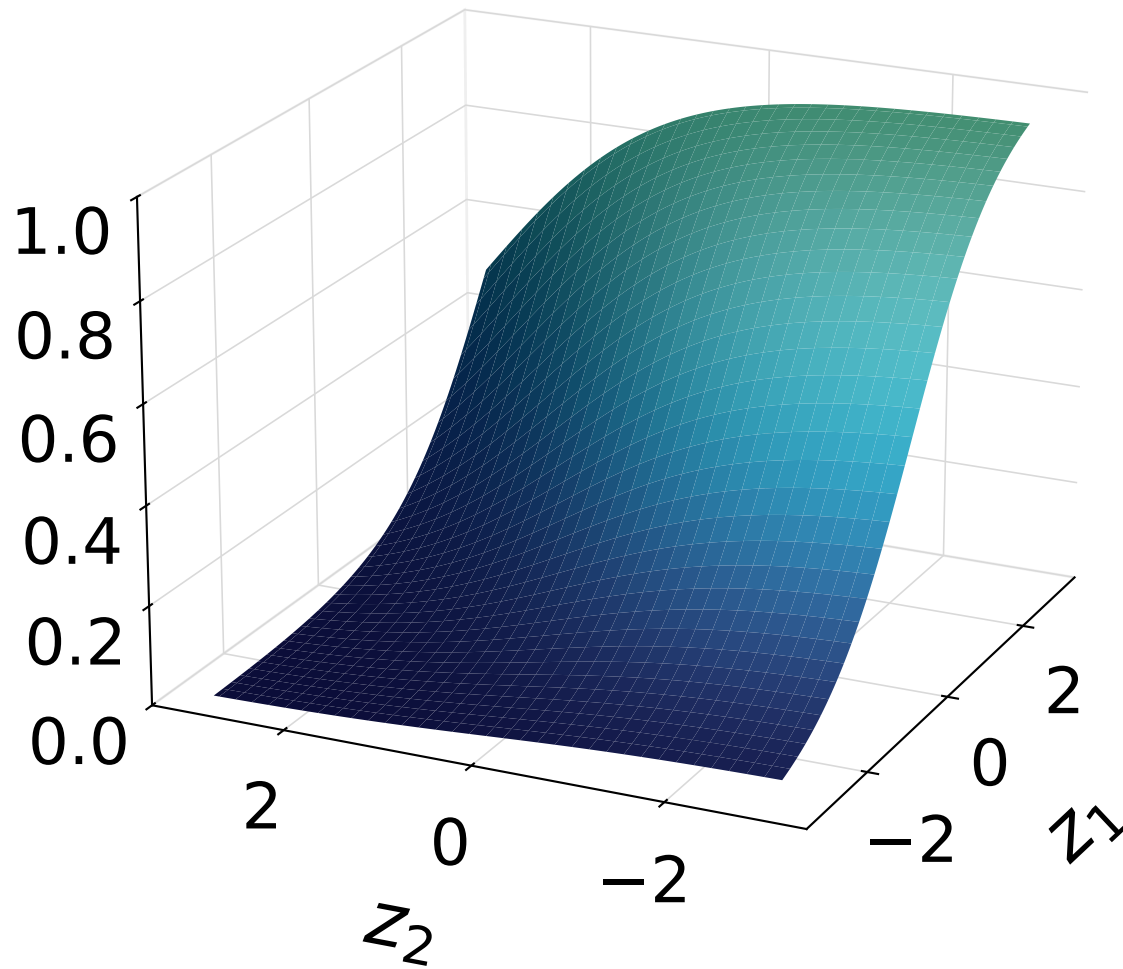
Softmax
