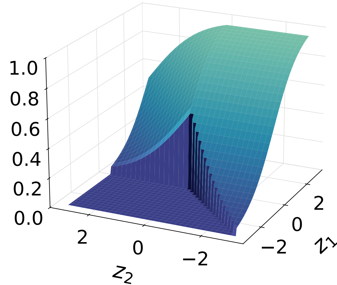
Top-2 softmax
