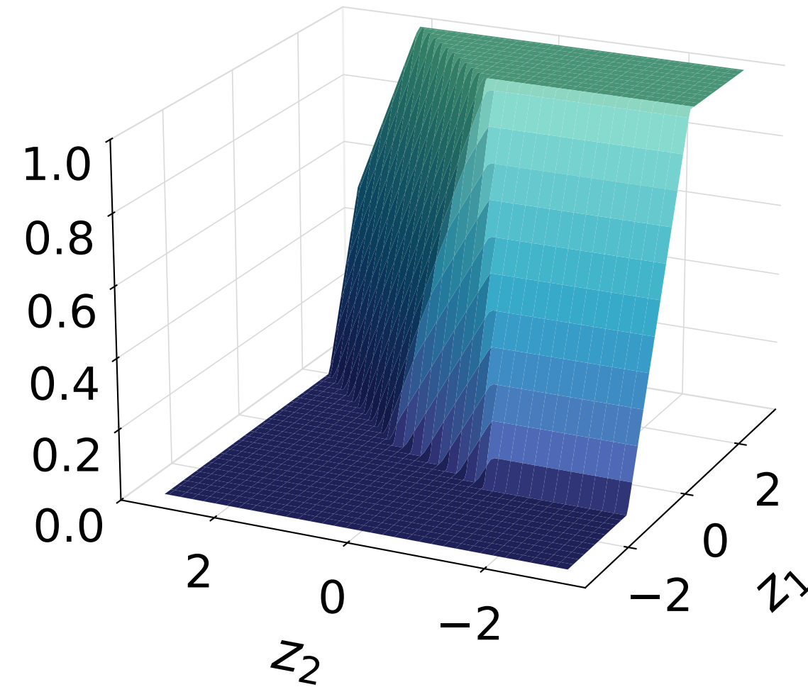
Sparsemax
