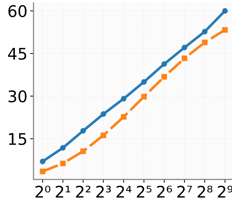
AIME25
