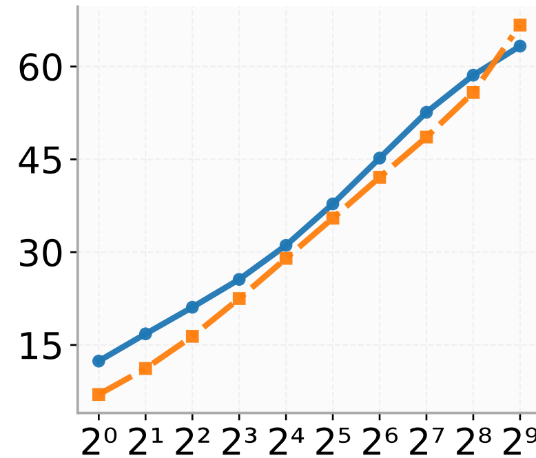
AIME24
