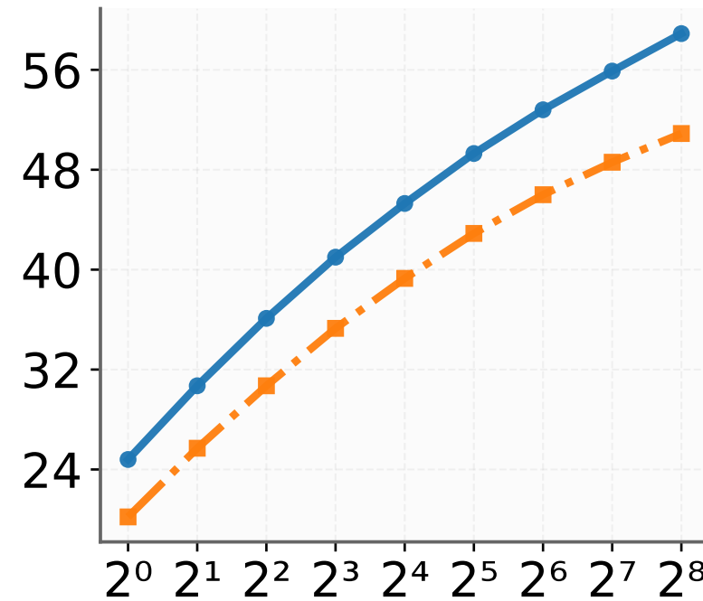
LiveCodeBench
