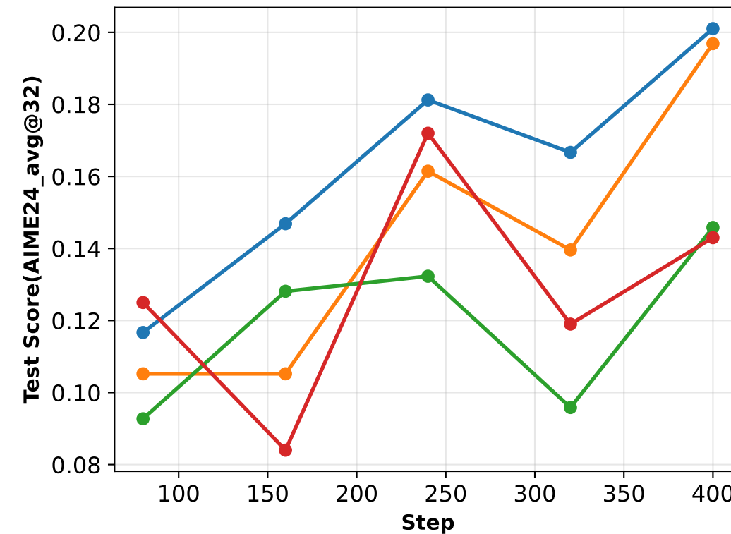
(d) Math Test
